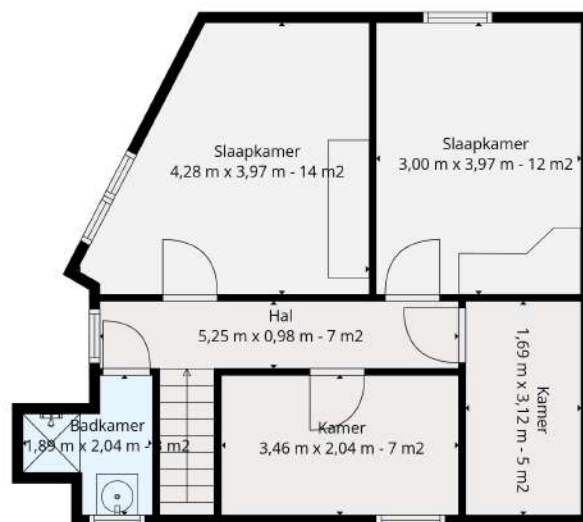
1e Verdieping
