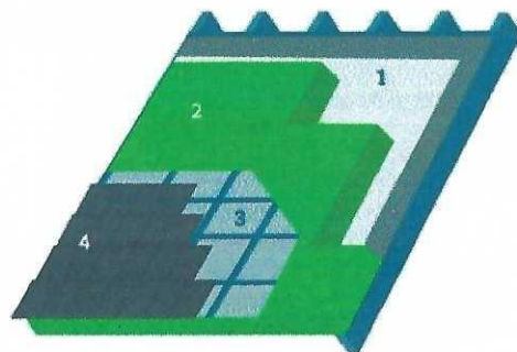
1. Dampscherm | 2. Isolatie | 3. Onderdak | 4. Dakbekleding
