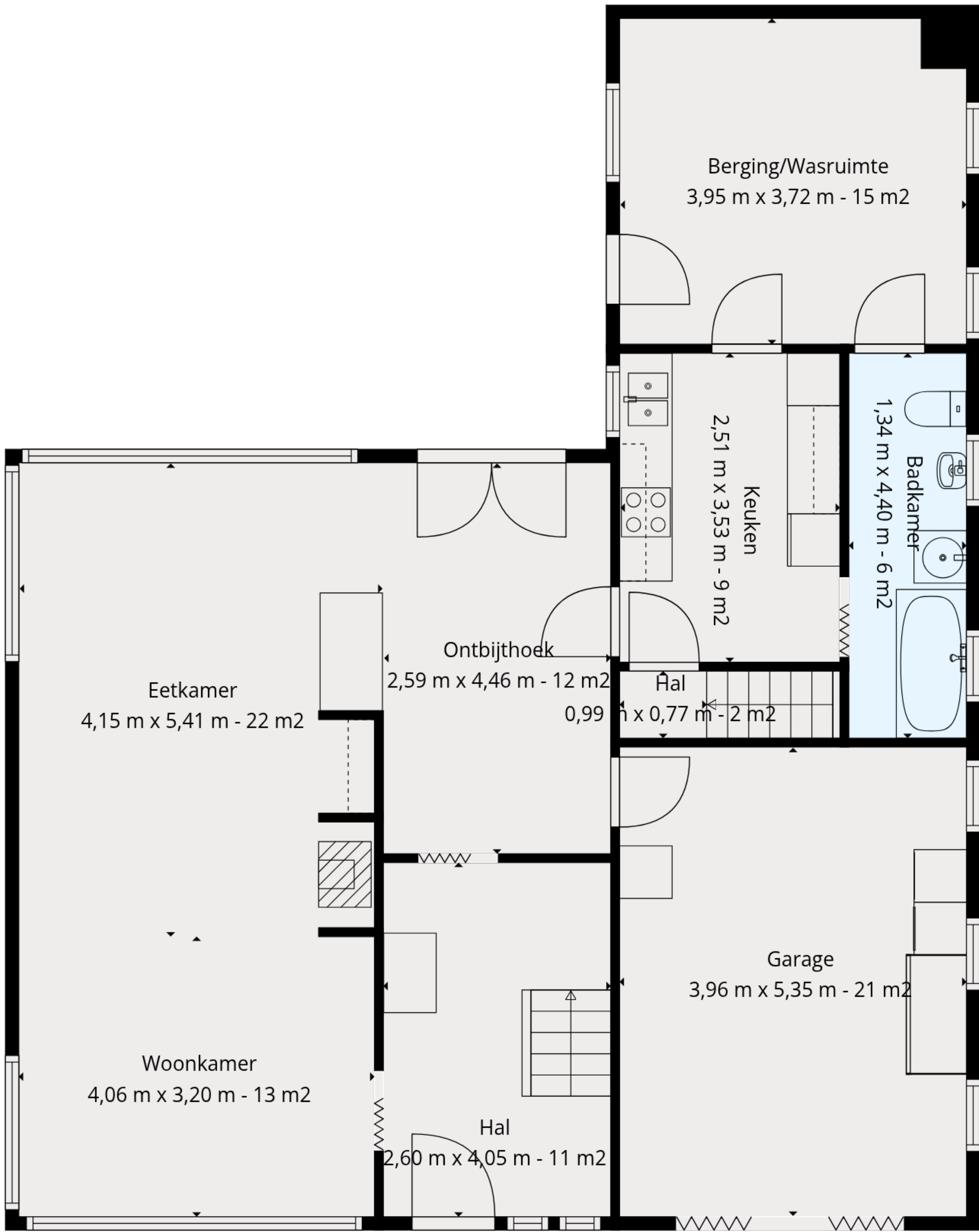
Gelijkvloerse Verdieping
