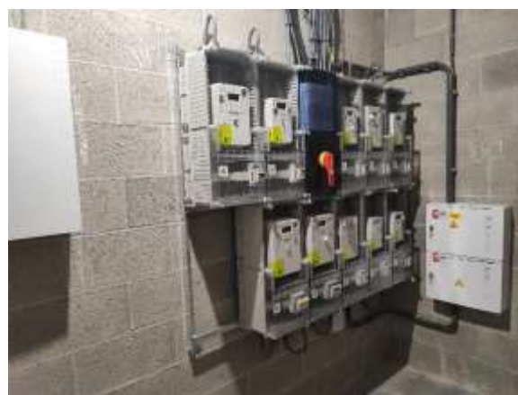
1 compteur électrique par appartements située dans le local technique bloc F
