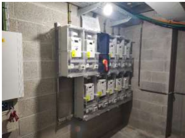
1 compteur électrique par appartements située dans le local technique bloc E
