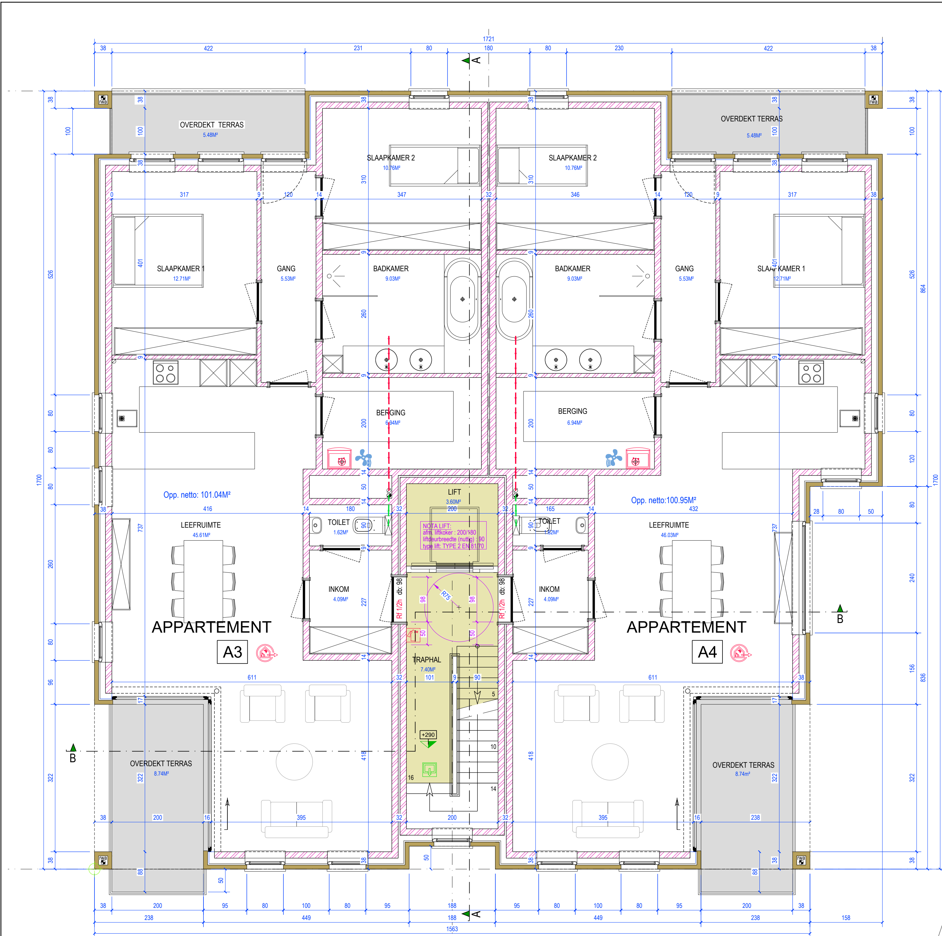
VERDIEPING 1
