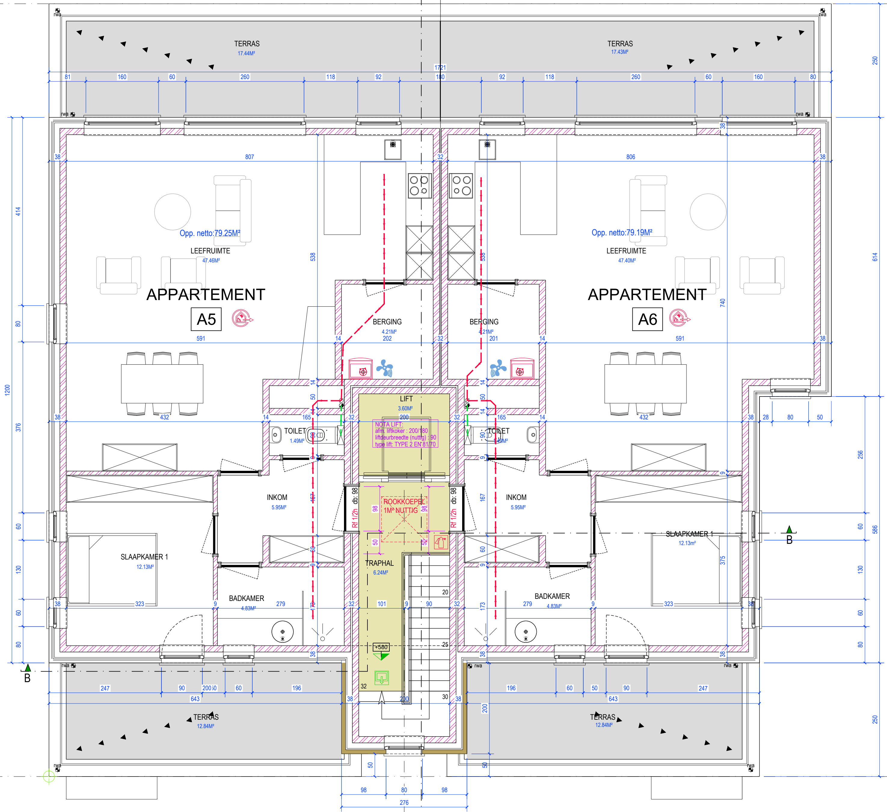
VERDIEPING 2
