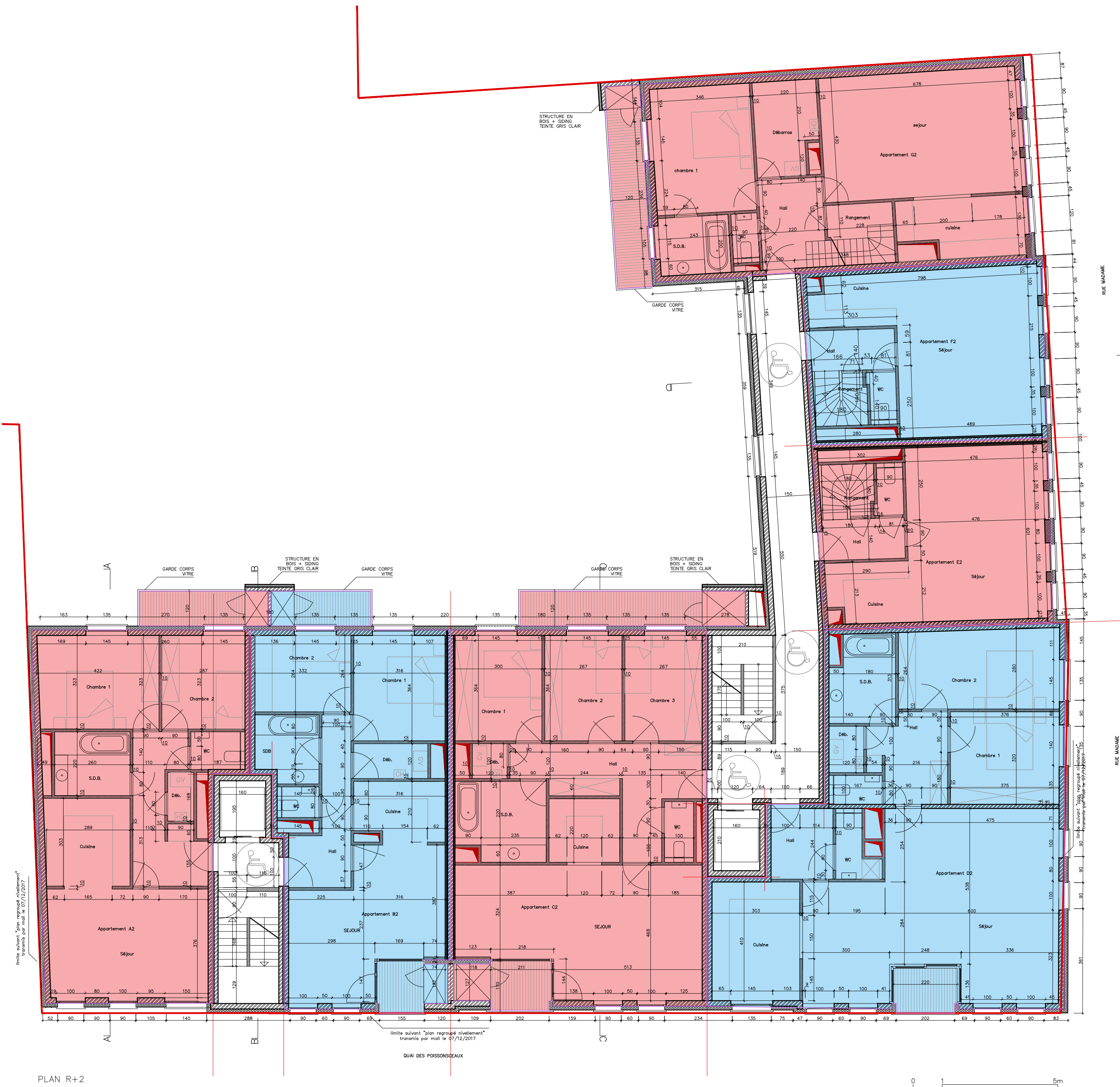
PLAN R+2
