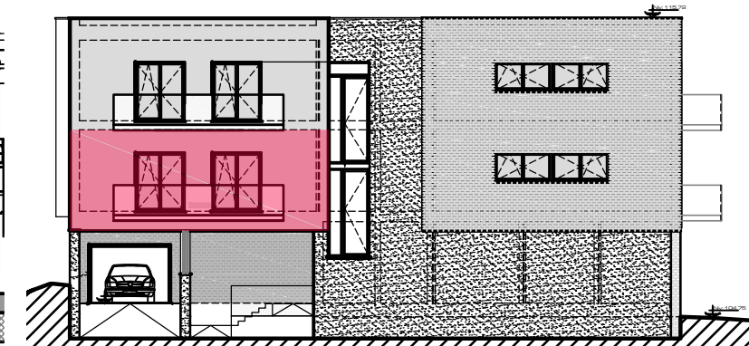
Situation projetée - Façade avant
