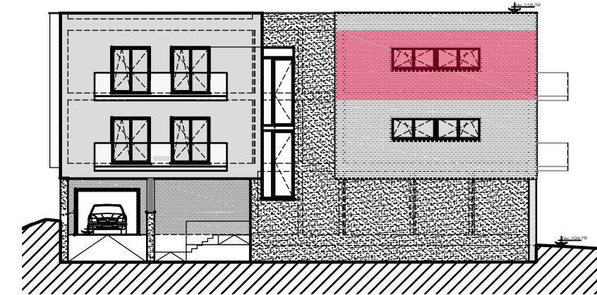
Situation projetée - Façade avant
