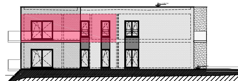
Situation projetée - Façade latérale droite
