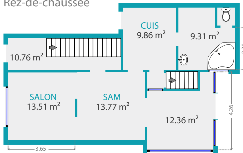
Rez-de-chaussée
