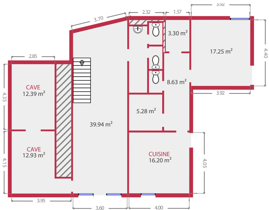
Rez-de-chaussée
