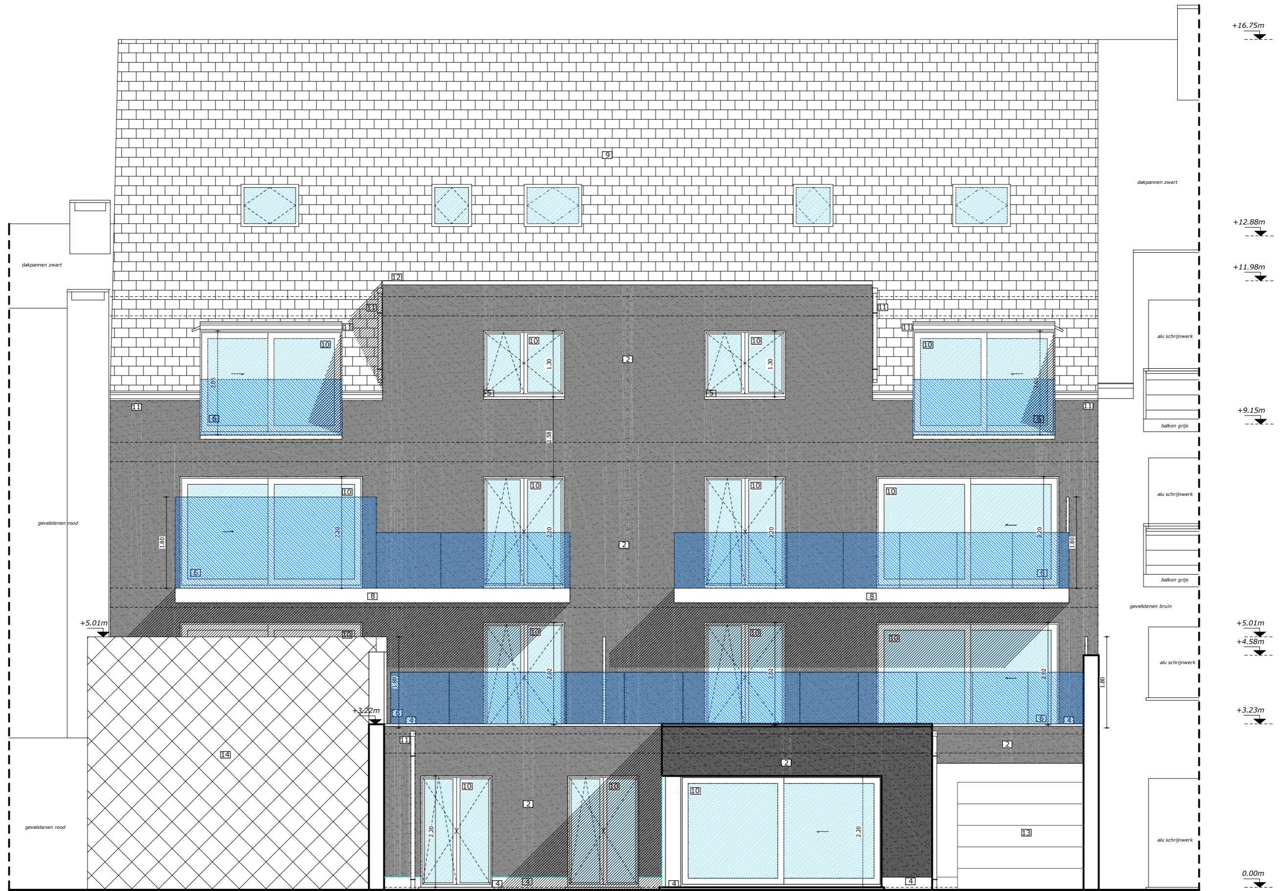
ACHTERGEVEL
