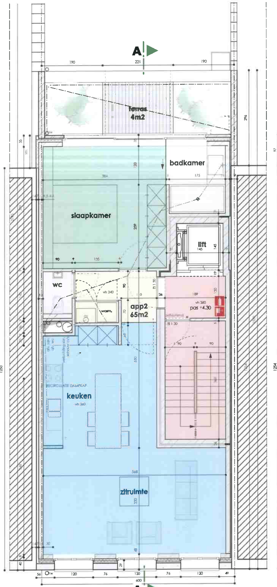
grondplan eerste verdieping 1/75
