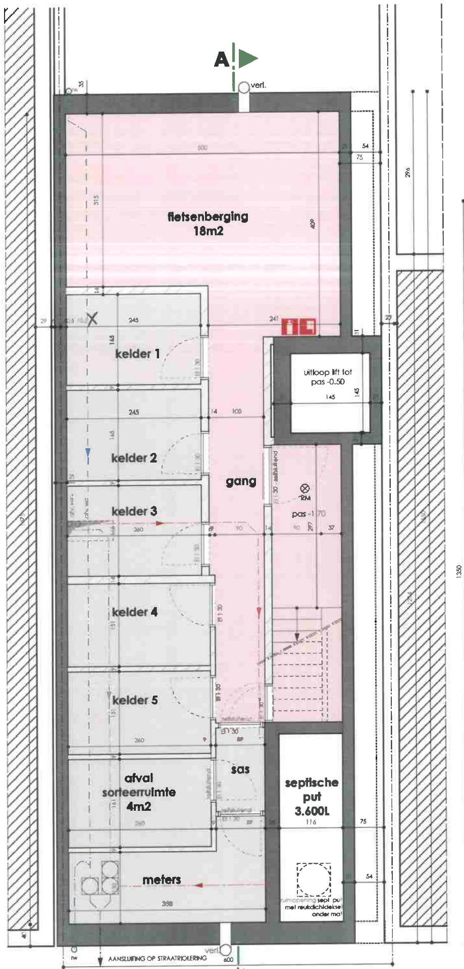
grondplan kelder 1/75
