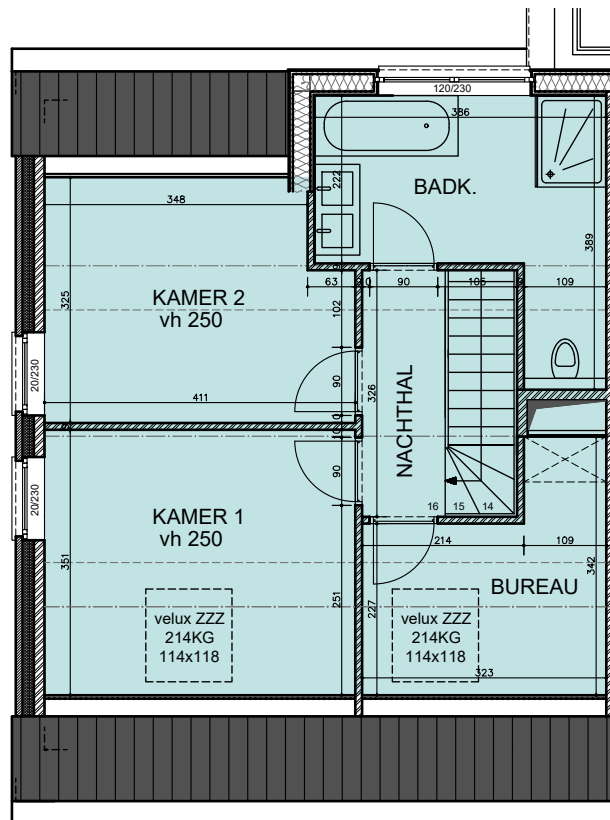
2de verdieping
