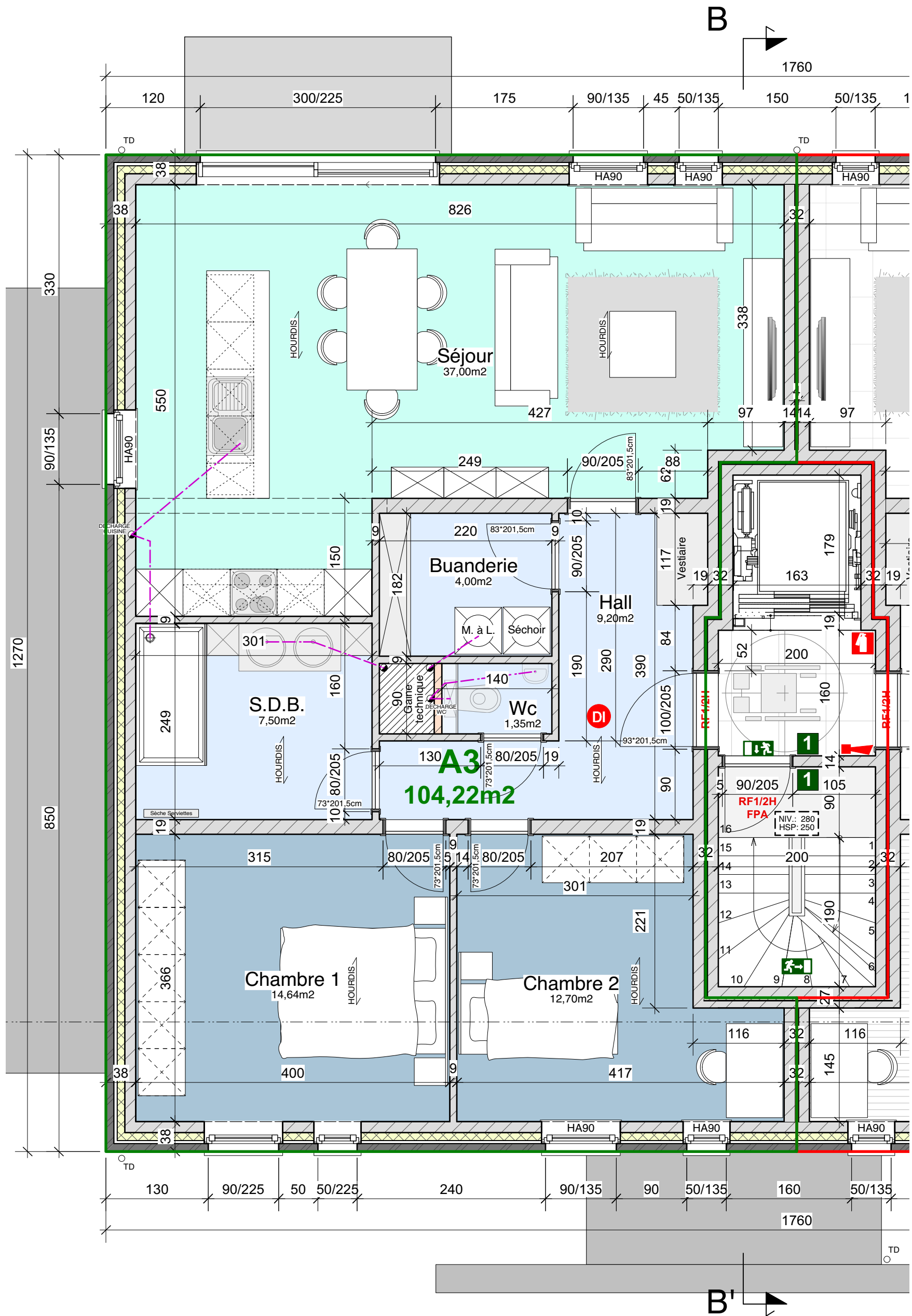
VUE EN PLAN DE L'ETAGE - APPARTEMENT 3
