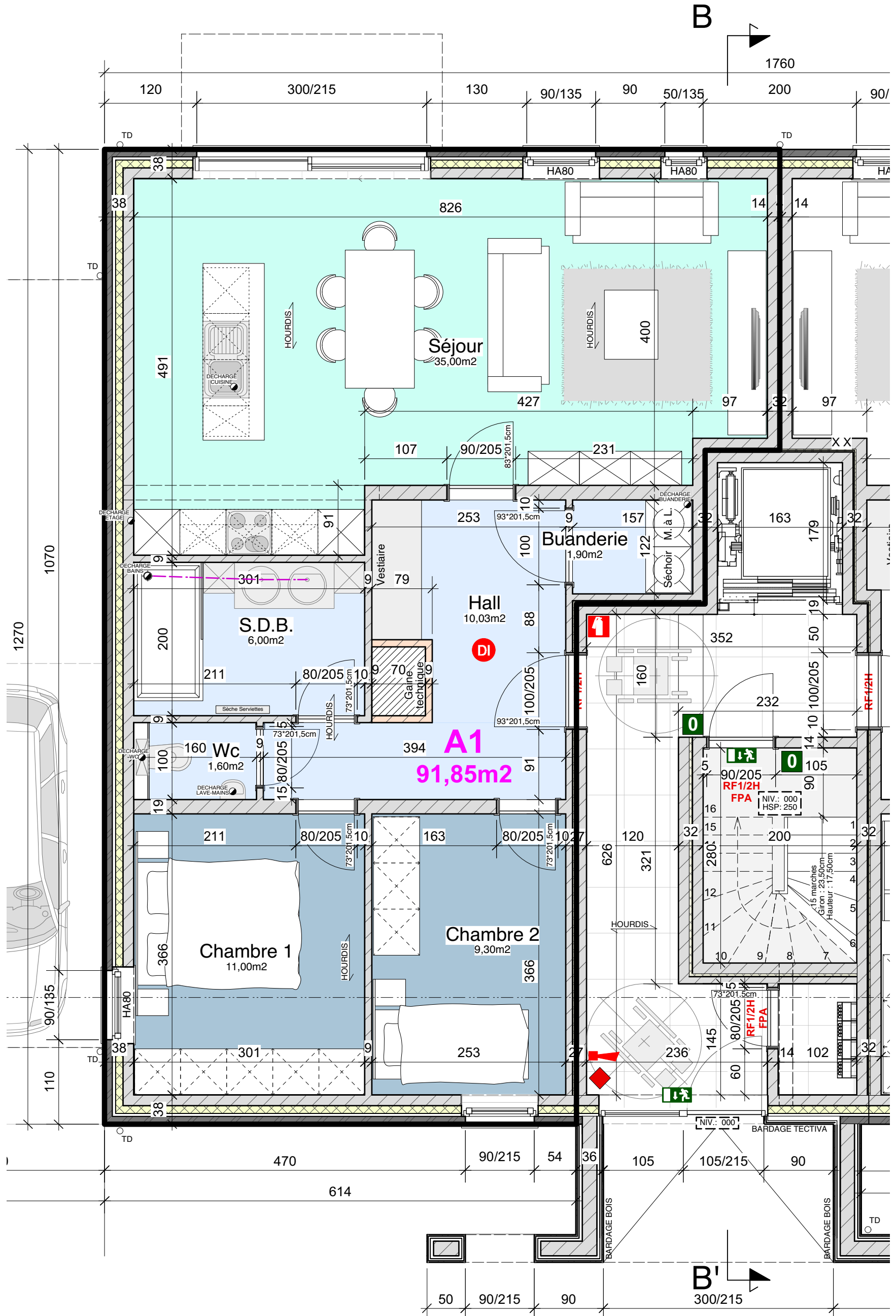
VUE EN PLAN DU REZ-DE-CHAUSSEE - APPARTEMENT 1
