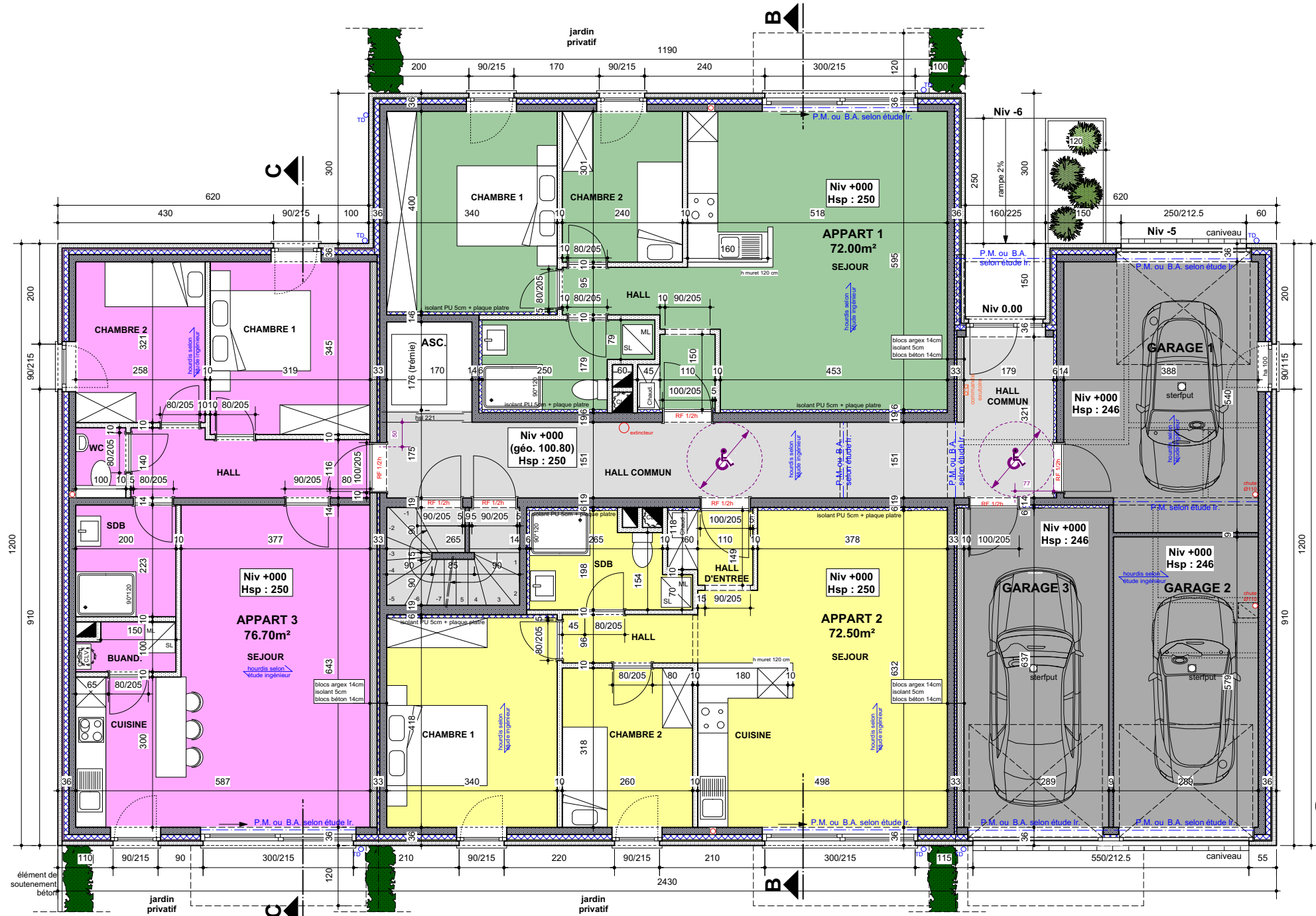
REZ (immeuble 2)
