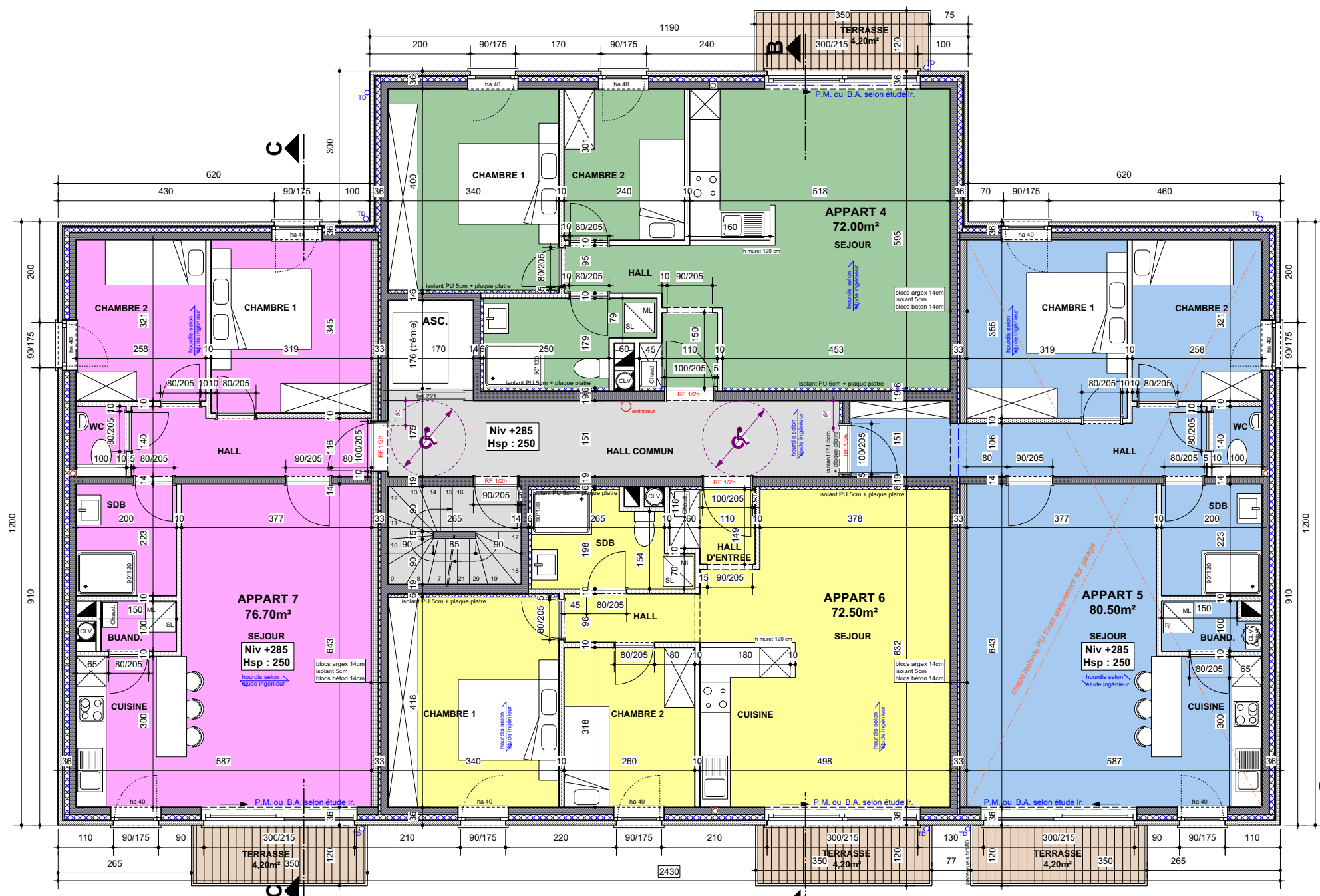
ETAGE 1 (immeuble 2)
