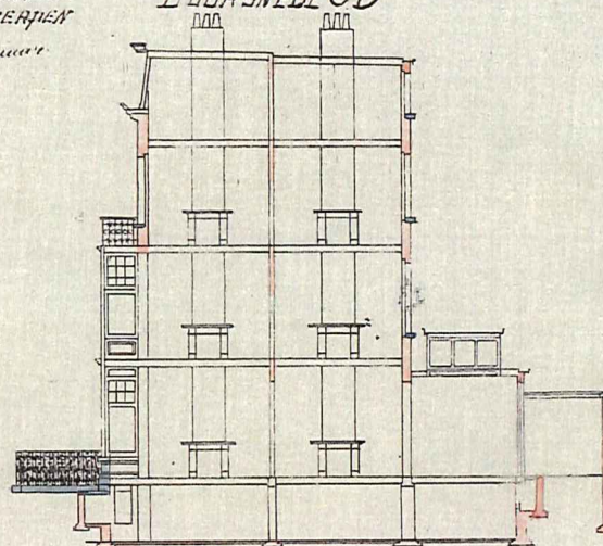
DOORSNEDE CD
