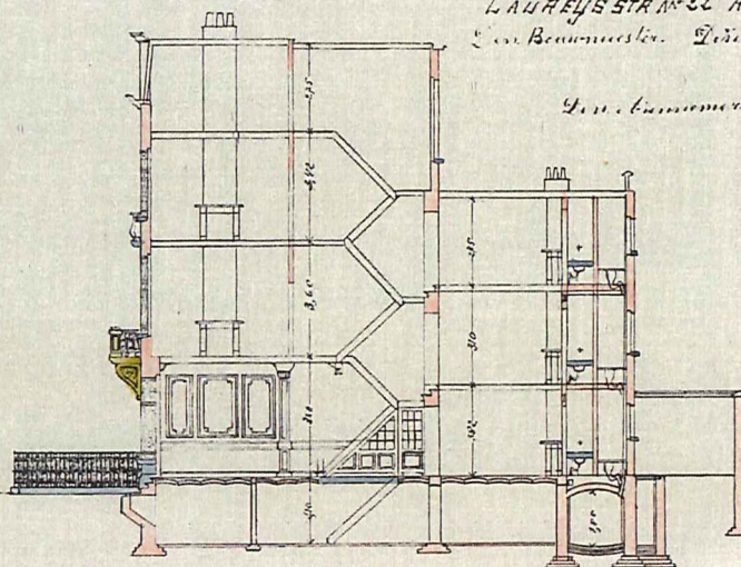
DOORSNEDE AB
