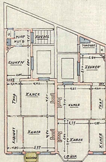
1 ste VERDIEPING
