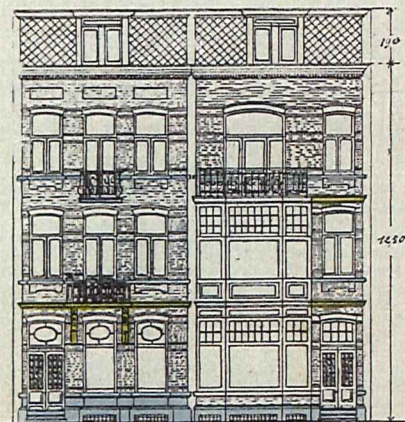
VOORGEVELS
