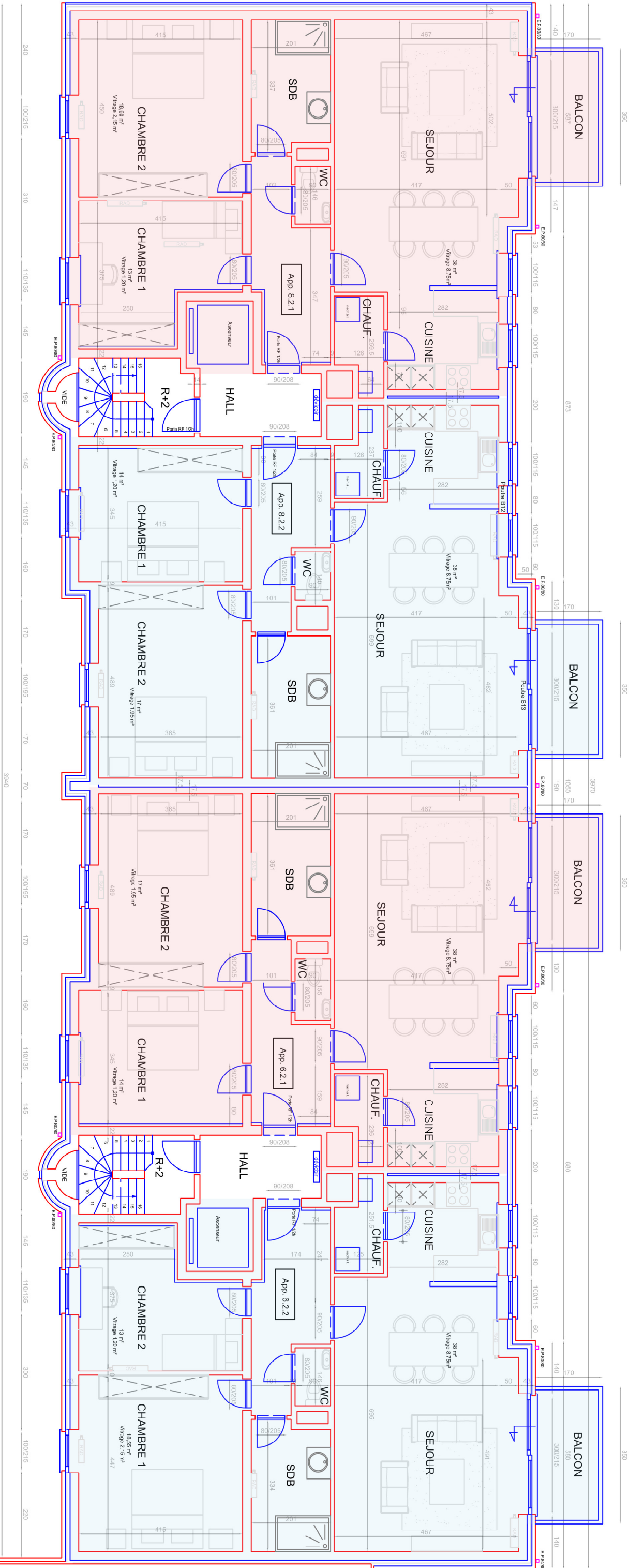
PLAN ETAGE 2
