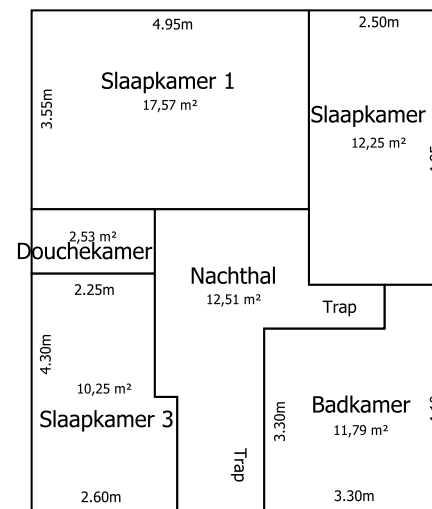
1ste verdieping
