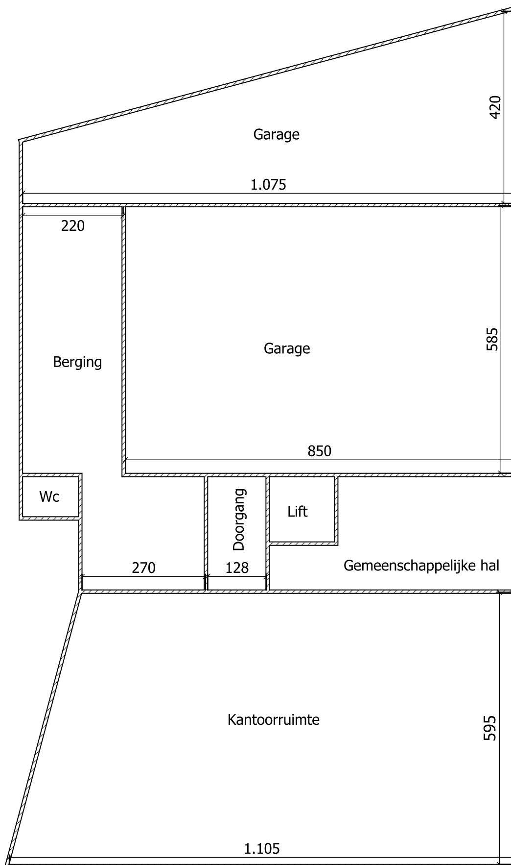
Gelijkvloers
