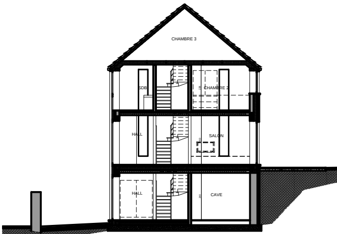
Coupe AA'
