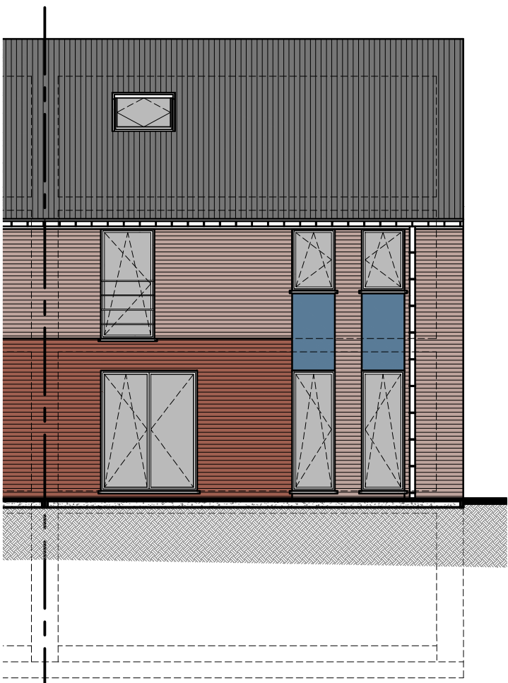
Elevation arrière
