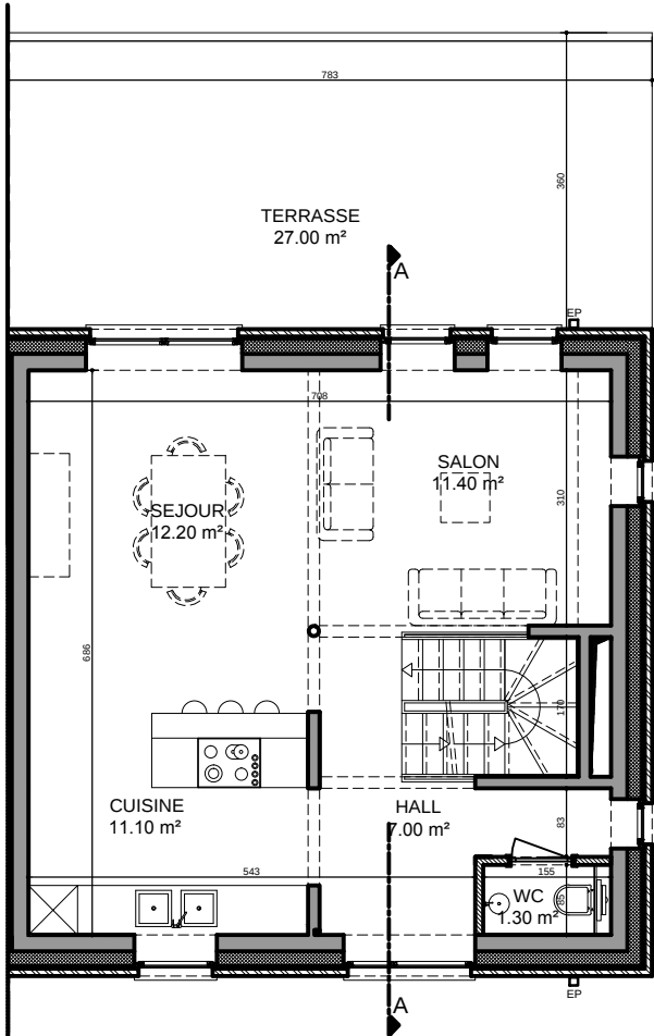
Rez-de-jardin
