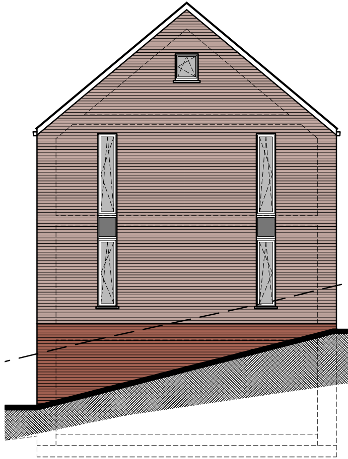
Elevation latérale
