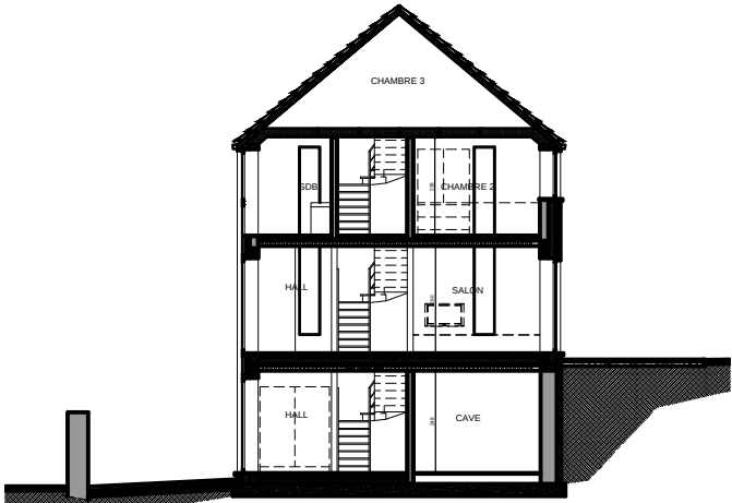
Coupe AA'
