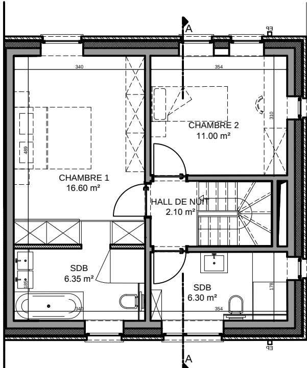
1er étage
