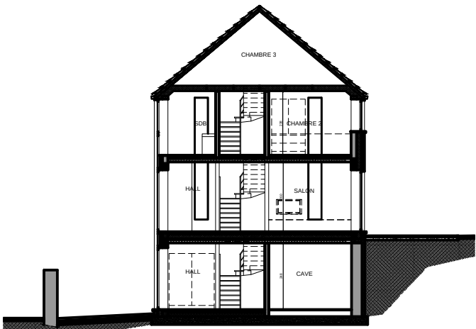
Coupe AA'
