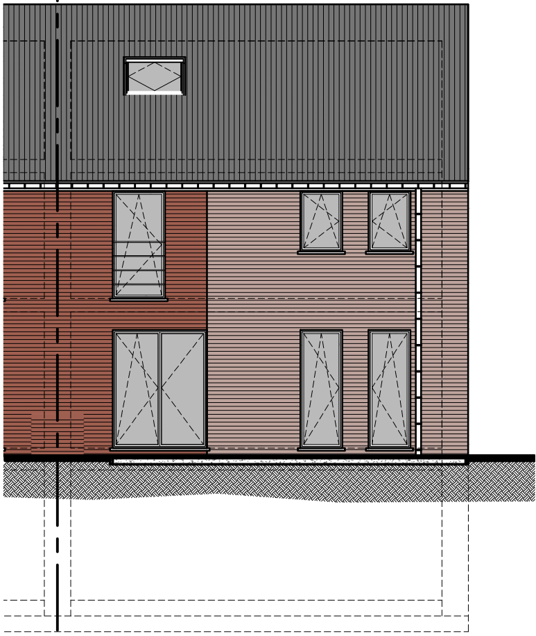
Elevation arrière
