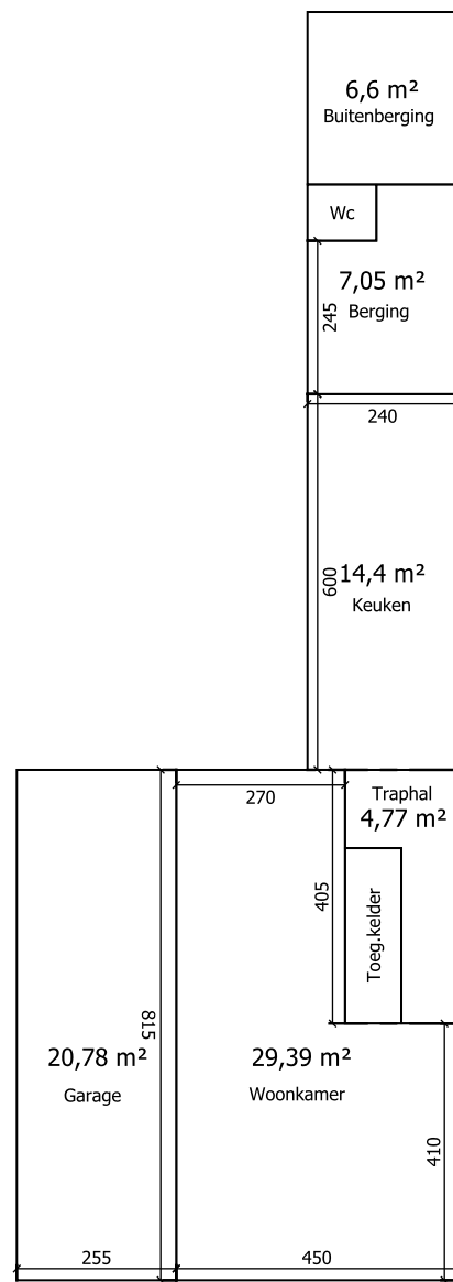
Gelijkvloers
