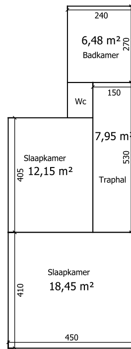
1ste verdieping
