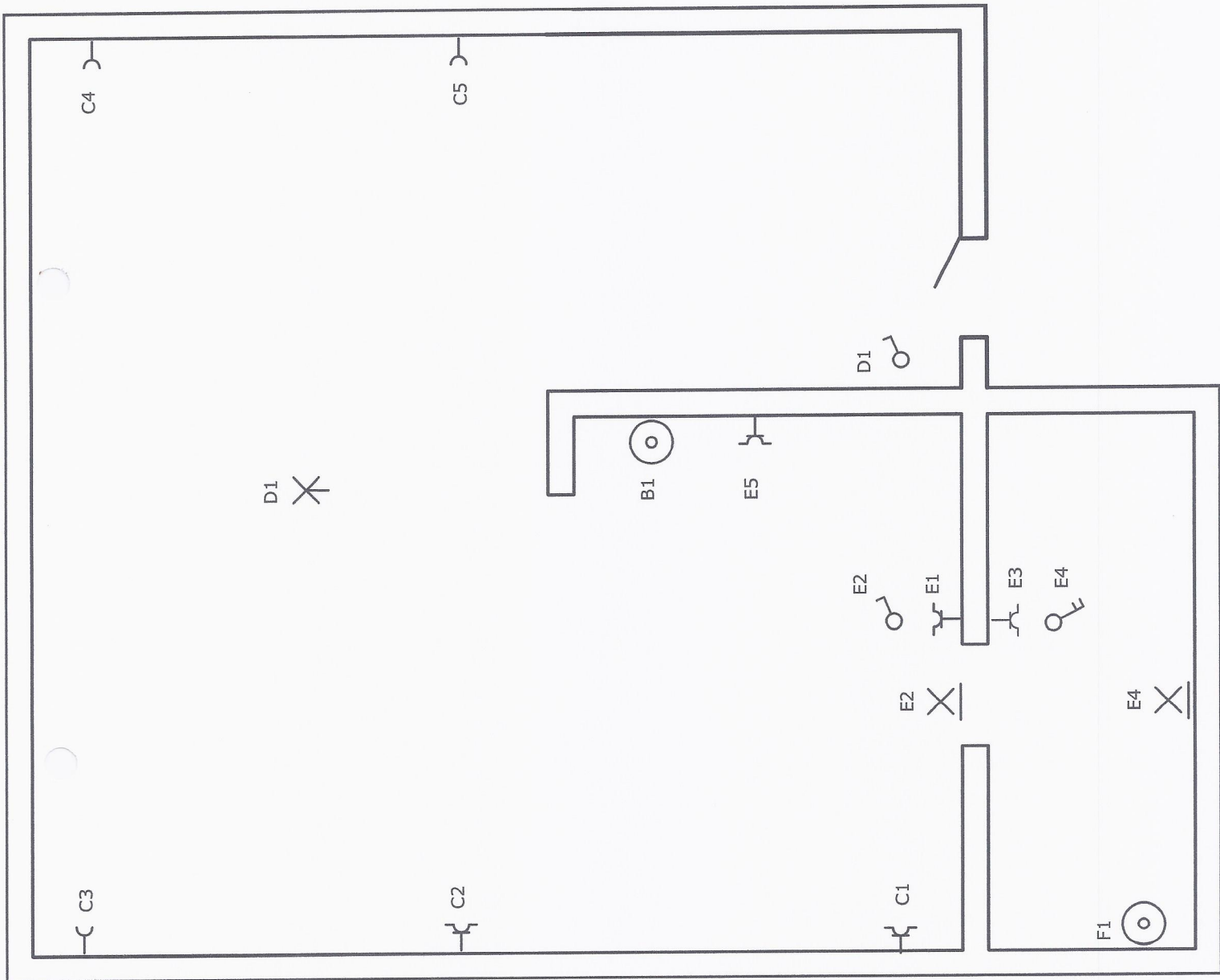
Situatieschema Greinstraat 66 1te ver. achter. 2060 Antwerpen.
