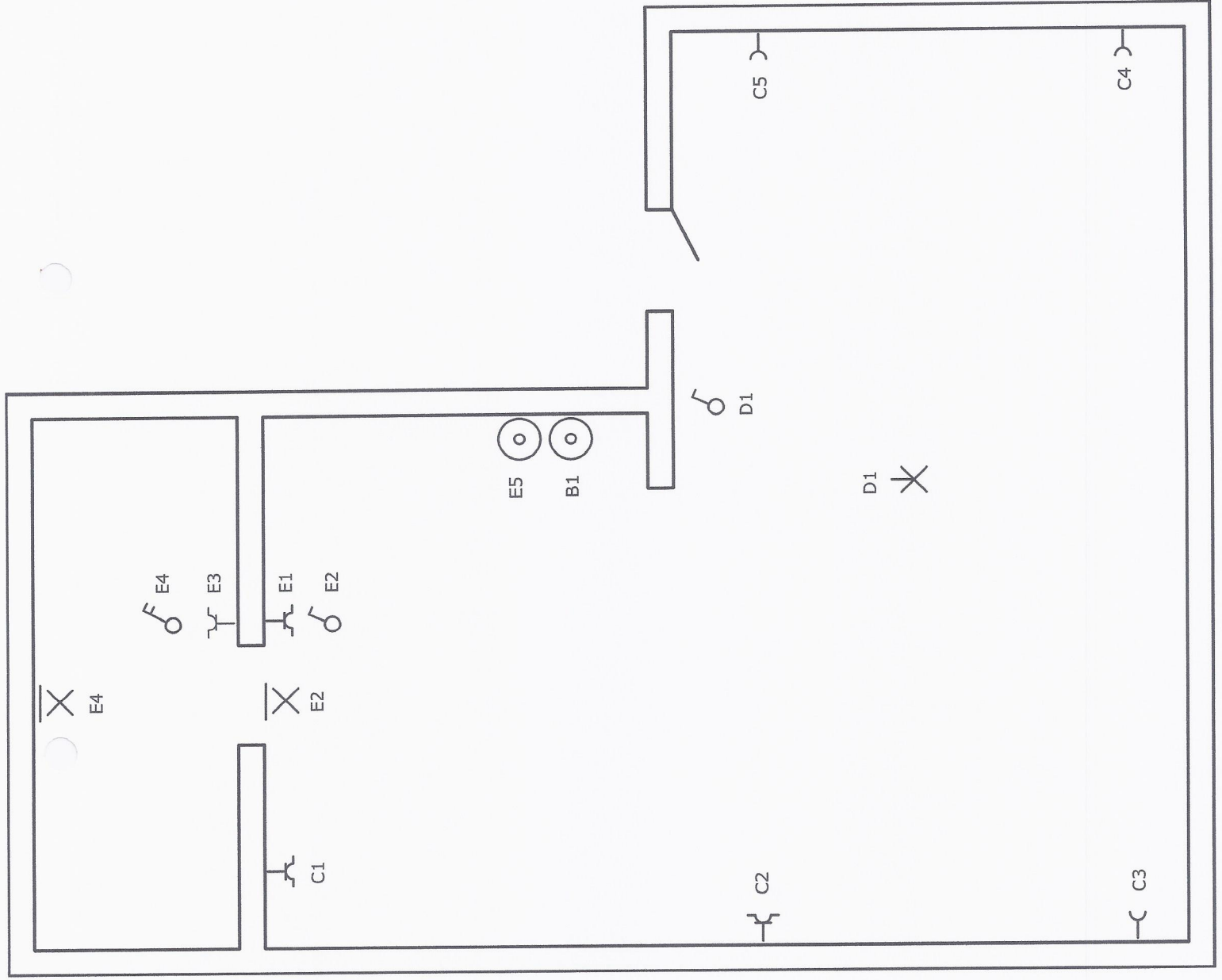
Situatieschema Greinstraat 66 1te ver. voor. 2060 Antwerpen.
