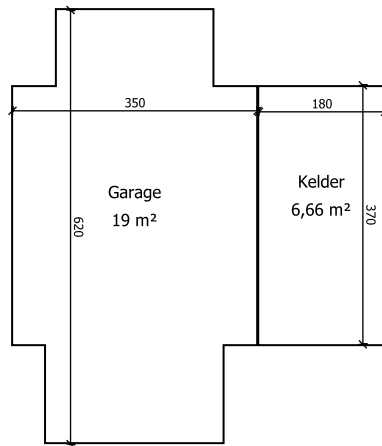
Kelderverdieping
