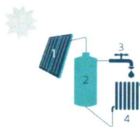
1 Zonnecollector | 2 Opslagvat zonnepanelen 3 Sanitair (bad, douche) water 4 Rooktelement voor ruimteverwarming 5 Opslagvat voor ruimteverwarming
