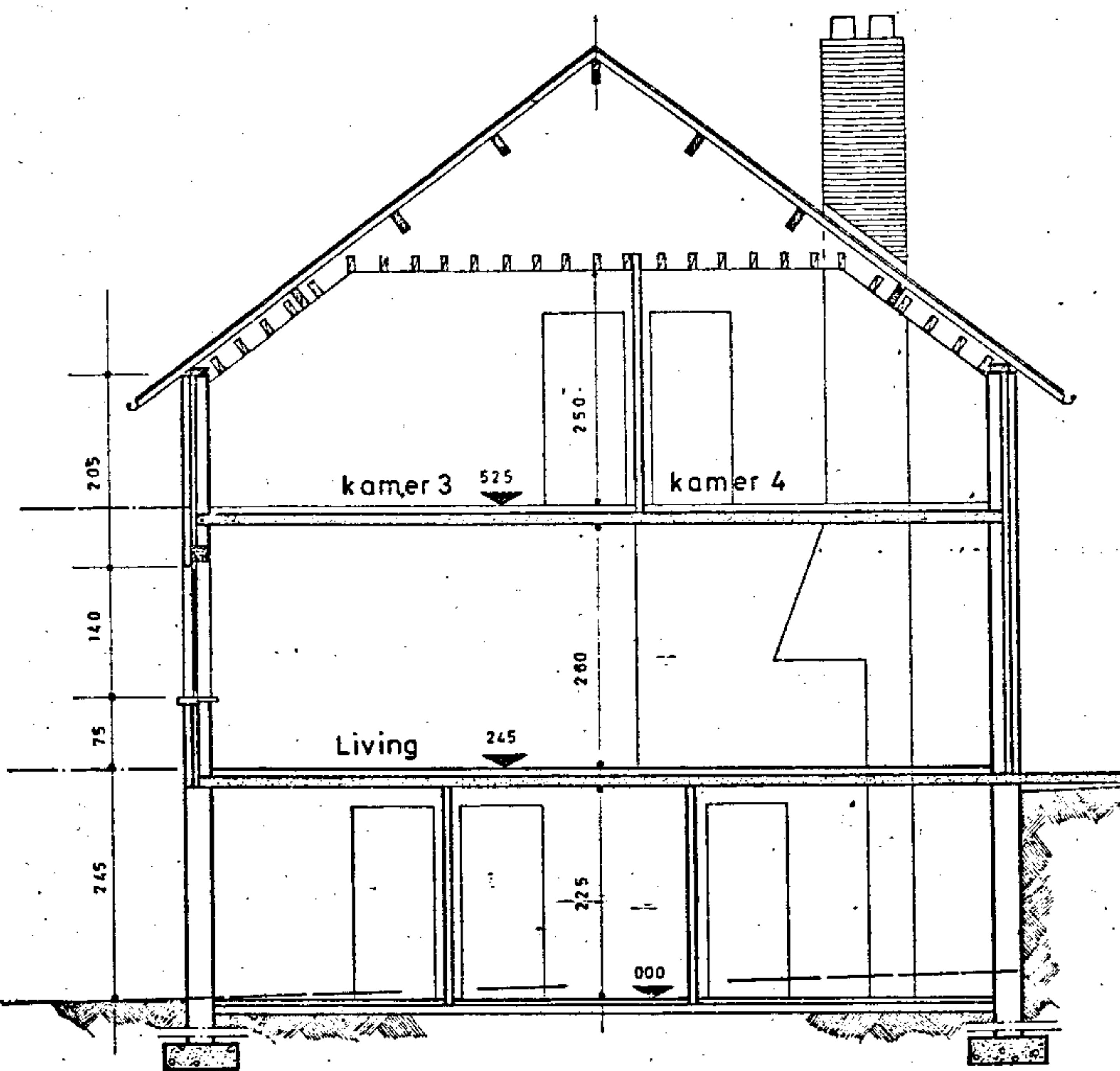
DOORSNEDE AB
