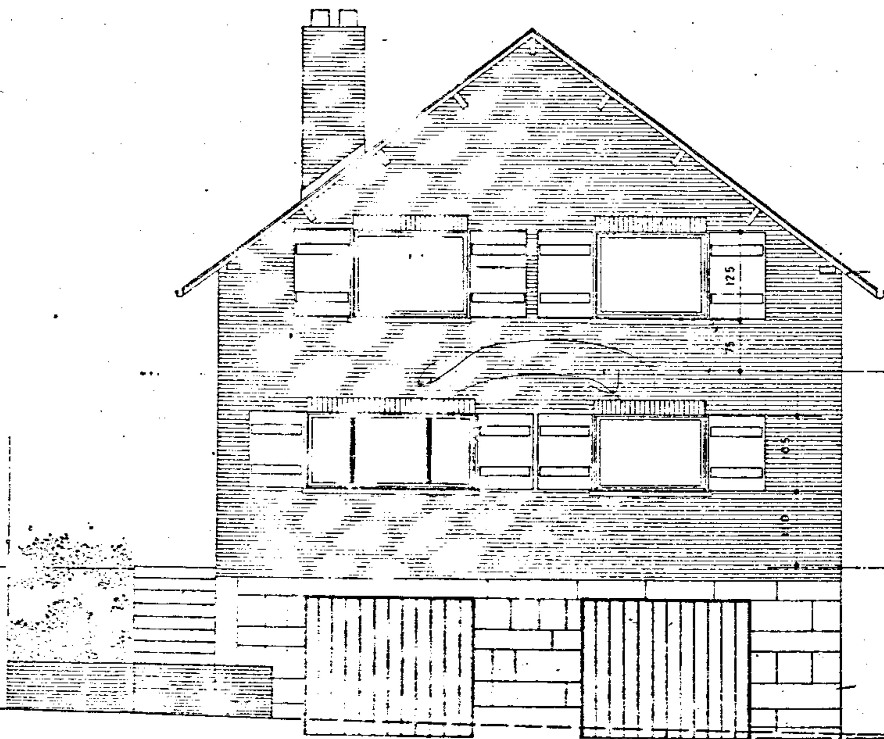
VOORGEVEL
