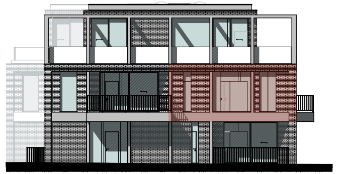
rechter zijgevel
