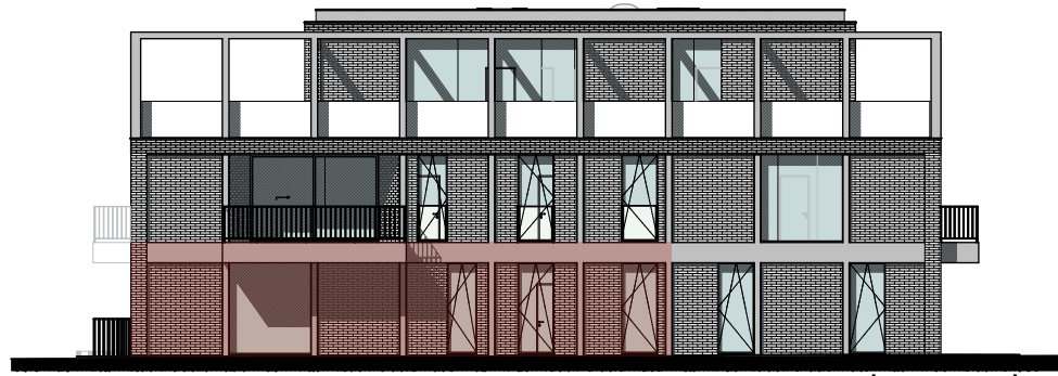
achtergevel
