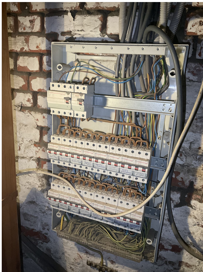
Verdeelborden 2
