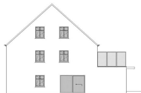
ZIJGEVEL RECHTS
