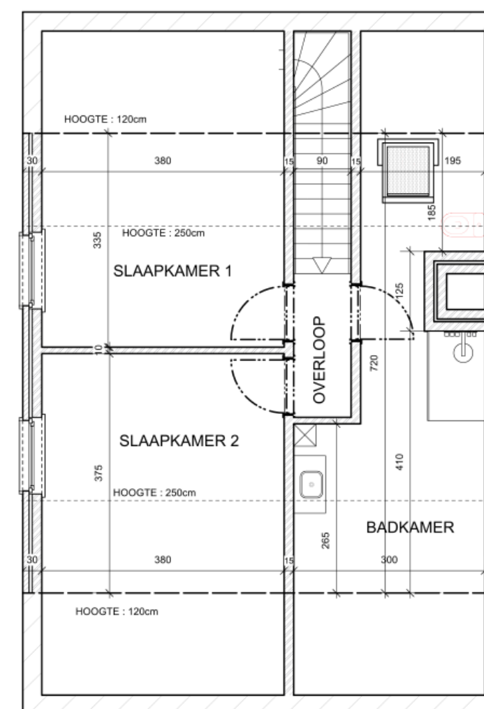
Slaapverdieping
