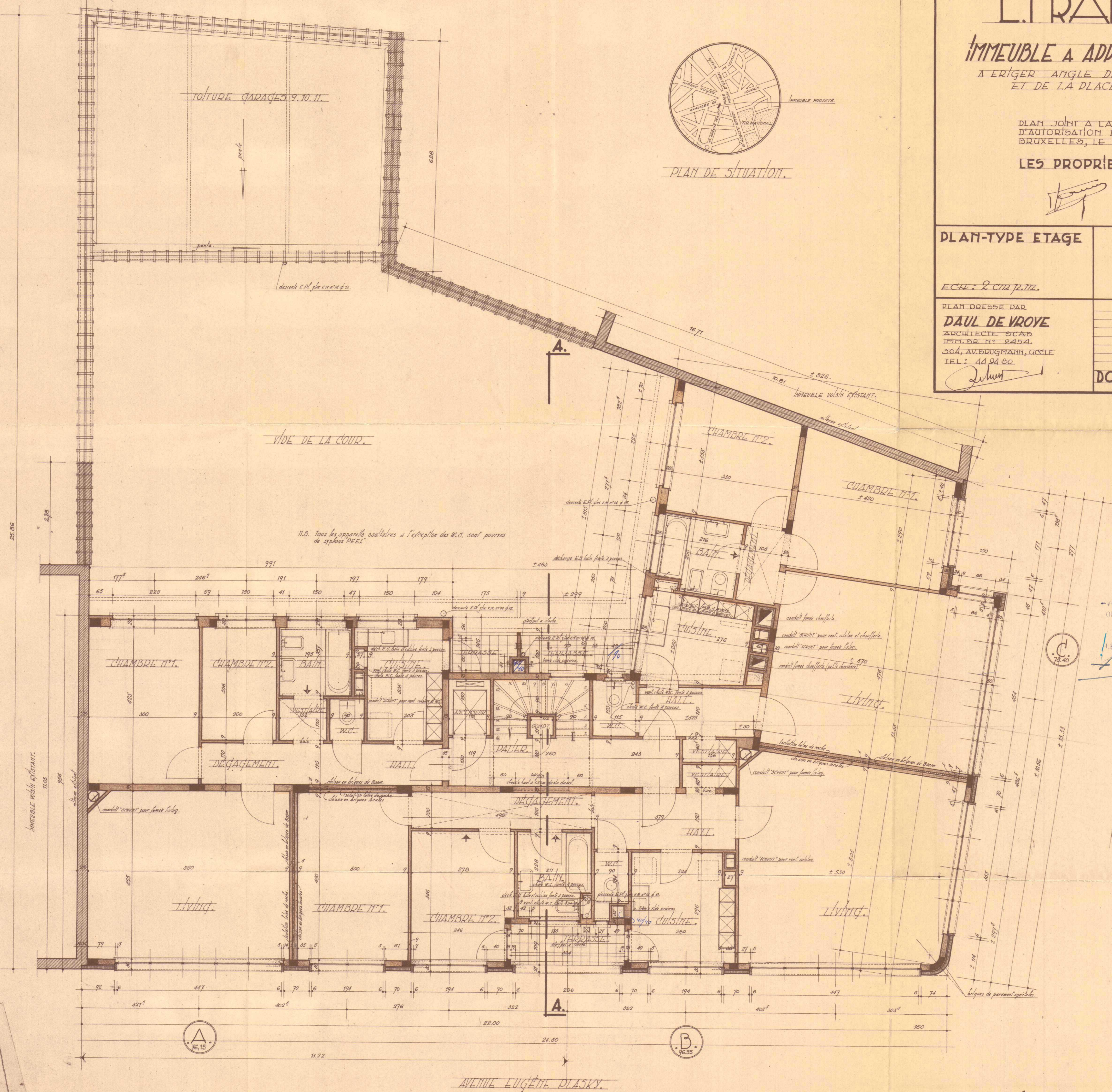
PLAN D'UN ÉTAGE TYPE
