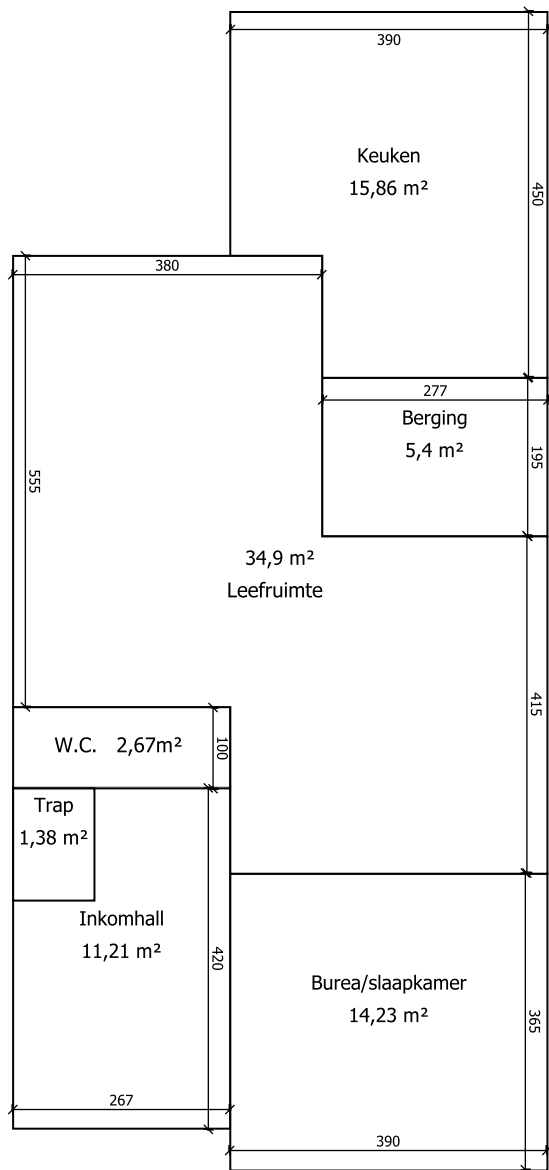
Gelijkvloers
