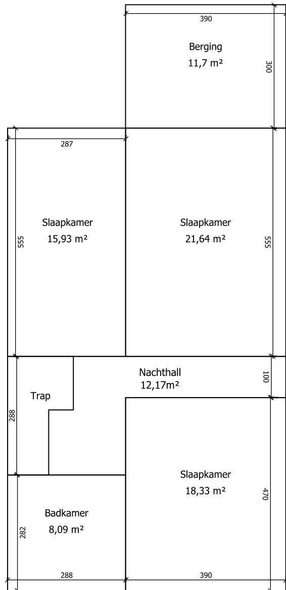
1ste verdieping
