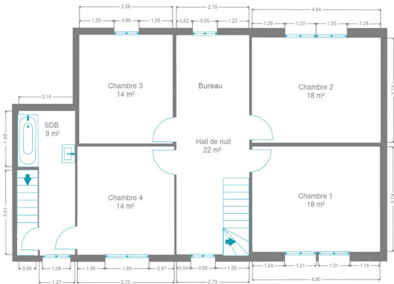
1er étage
