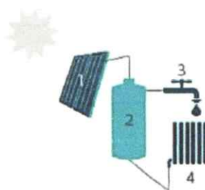
1 Zonnecollector | 2 Opslagvat zonneboiler | 3 Sanitair warm water tap 4 Radiator voor ruimteverwarming (op voorraad)
