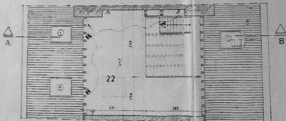
COMBLES : QUATRIEME ETAGE
