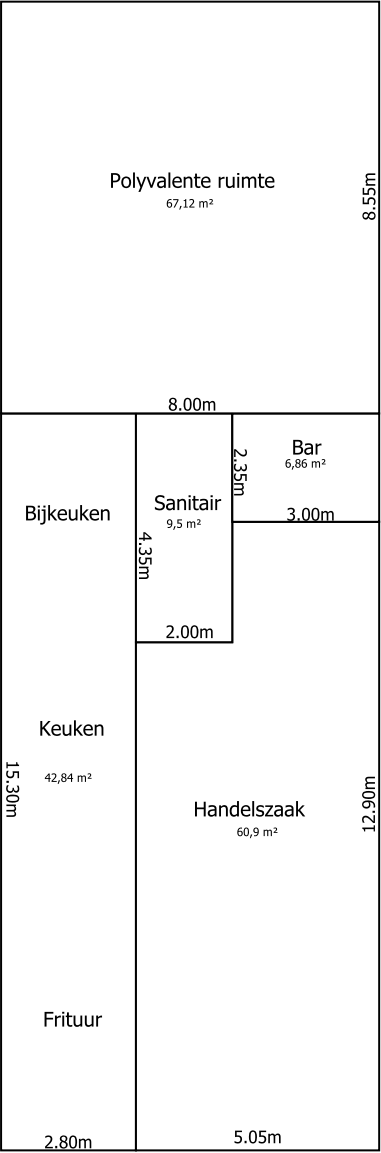
Gelijkvloers
