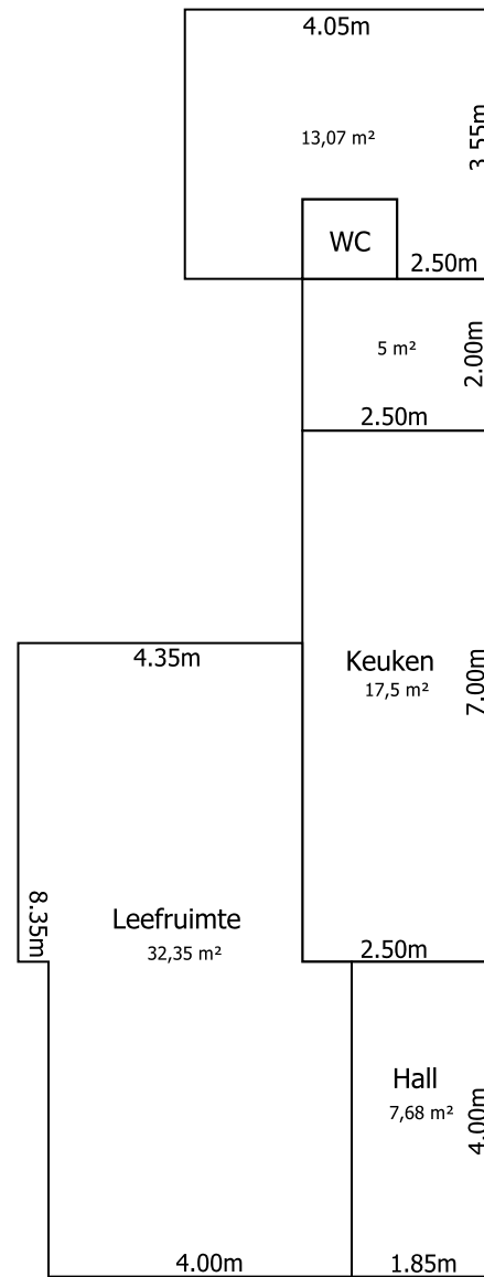
Gelijkvloers
