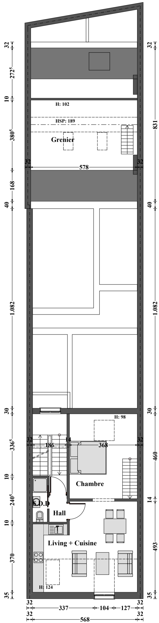
PLAN DES MANSARDES Echelle 1/100
