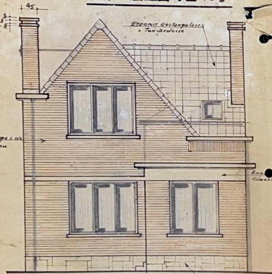
FAÇADE POSTÉRIEURE.
