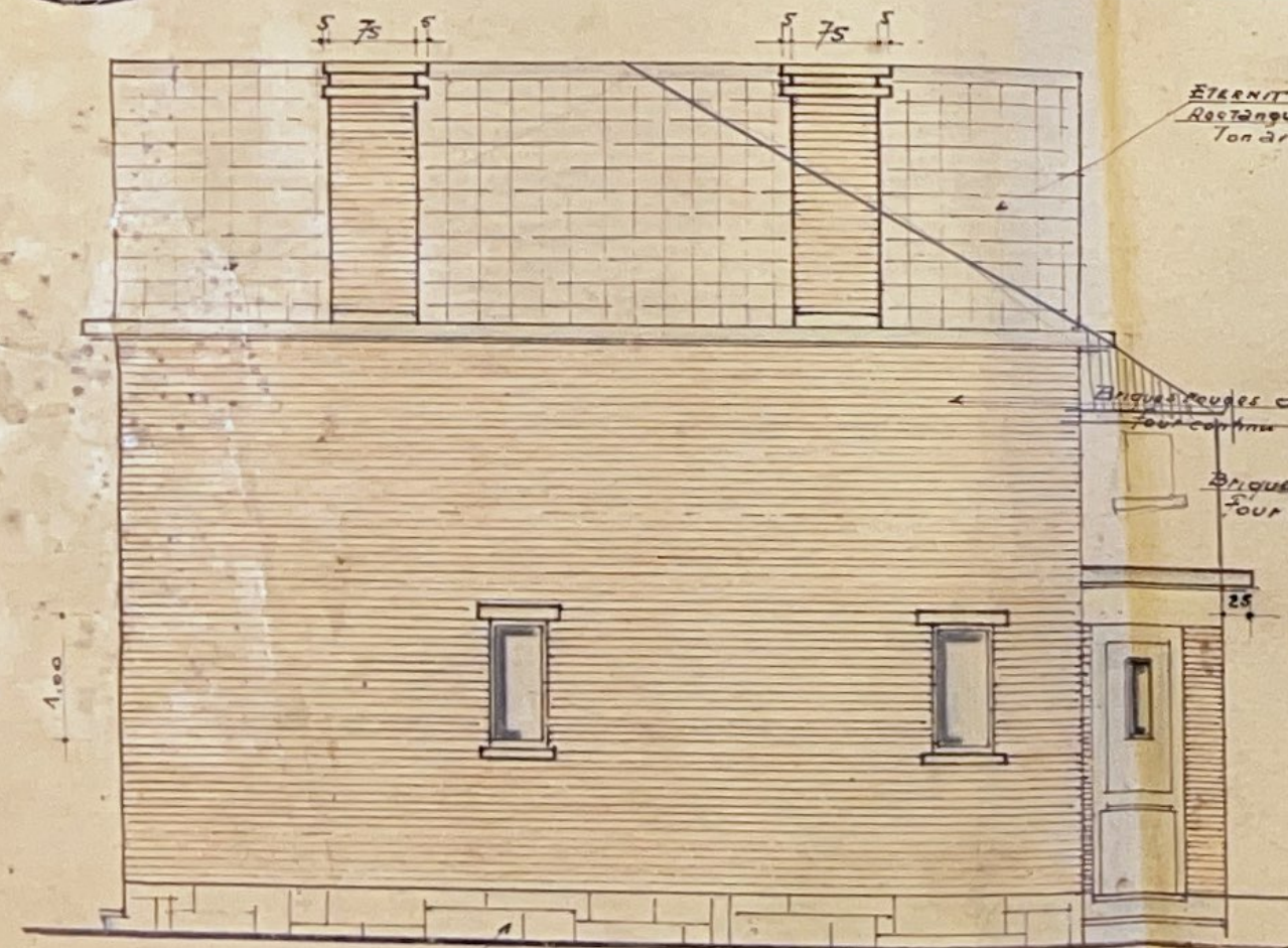
FAÇADE DROITE.
