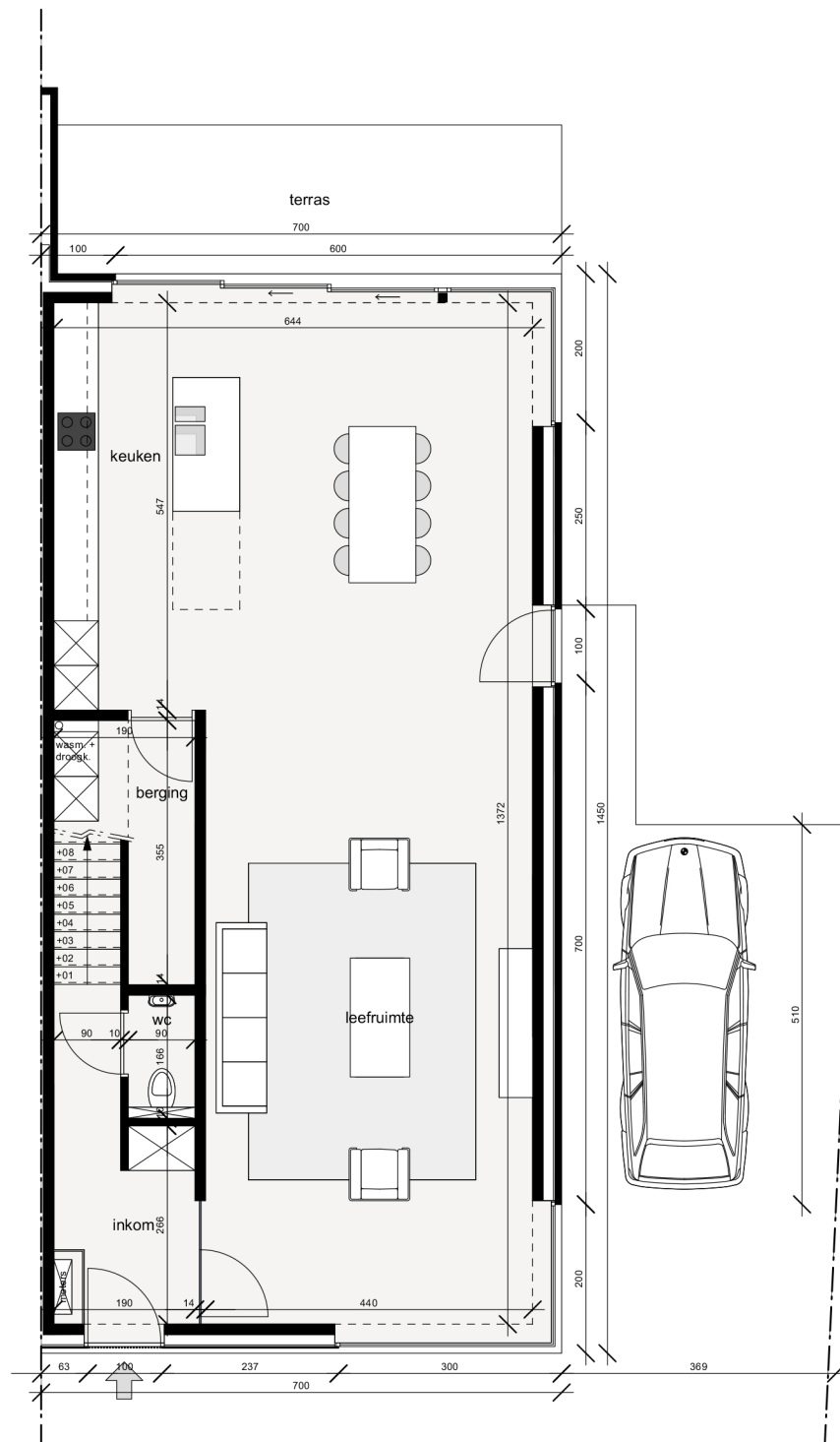
GELIJKVLOERS
