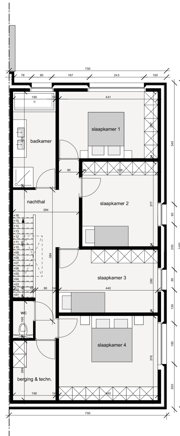
VERDIEPING
