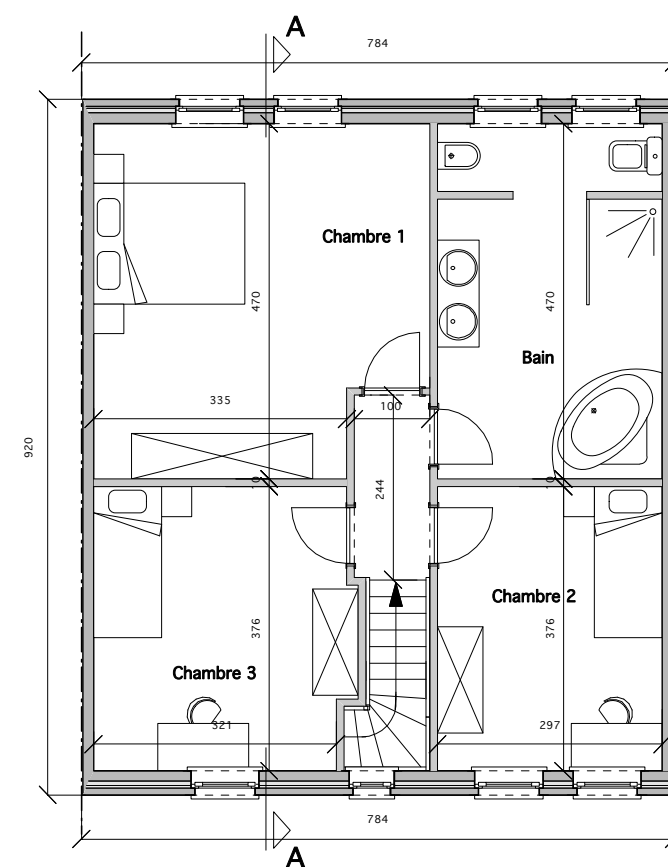
VUE EN PLAN ETAGE
