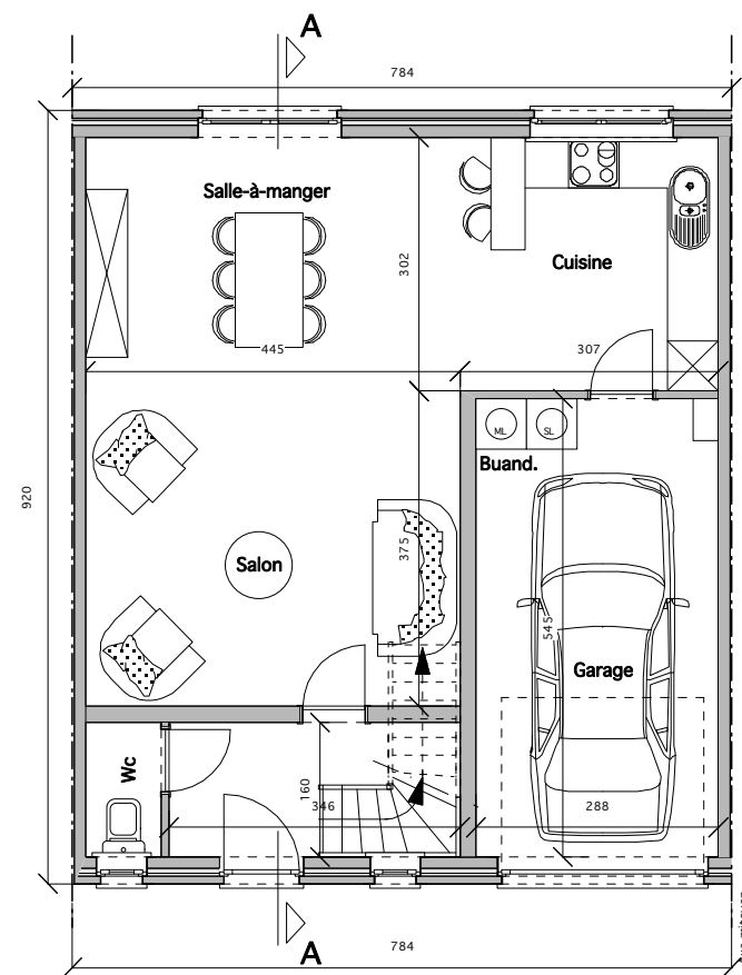
VUE EN PLAN REZ-DE-CHAUSSEE
