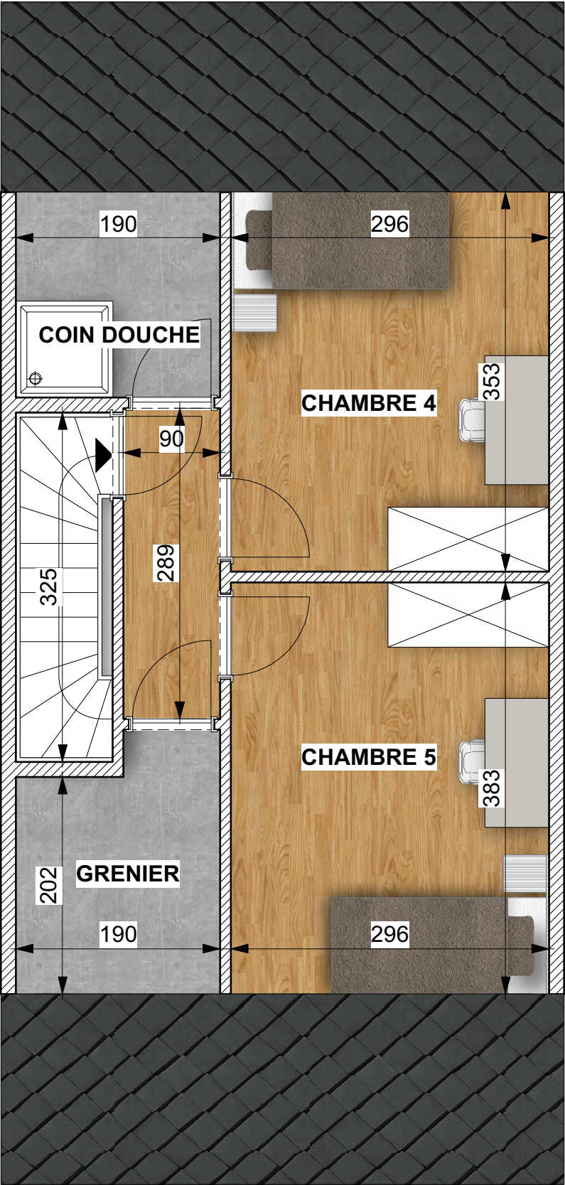
Maison M3 - PLAN DEUXIEME ETAGE
