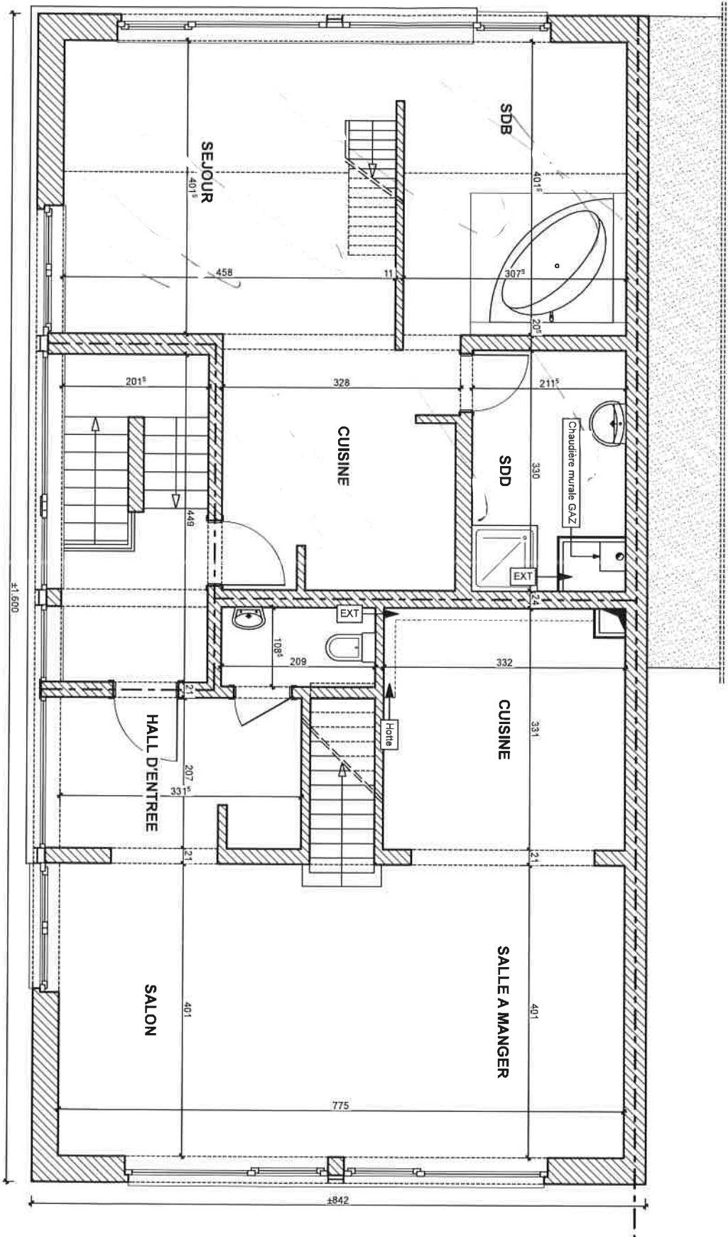
ETAGE 2 - 1/50
