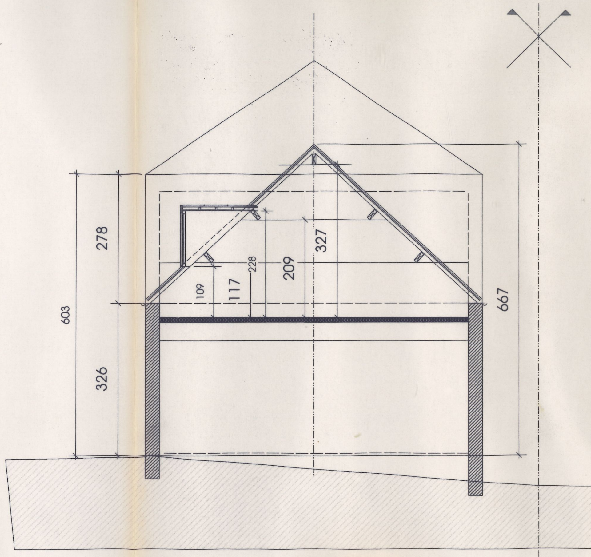
Coupe bb
