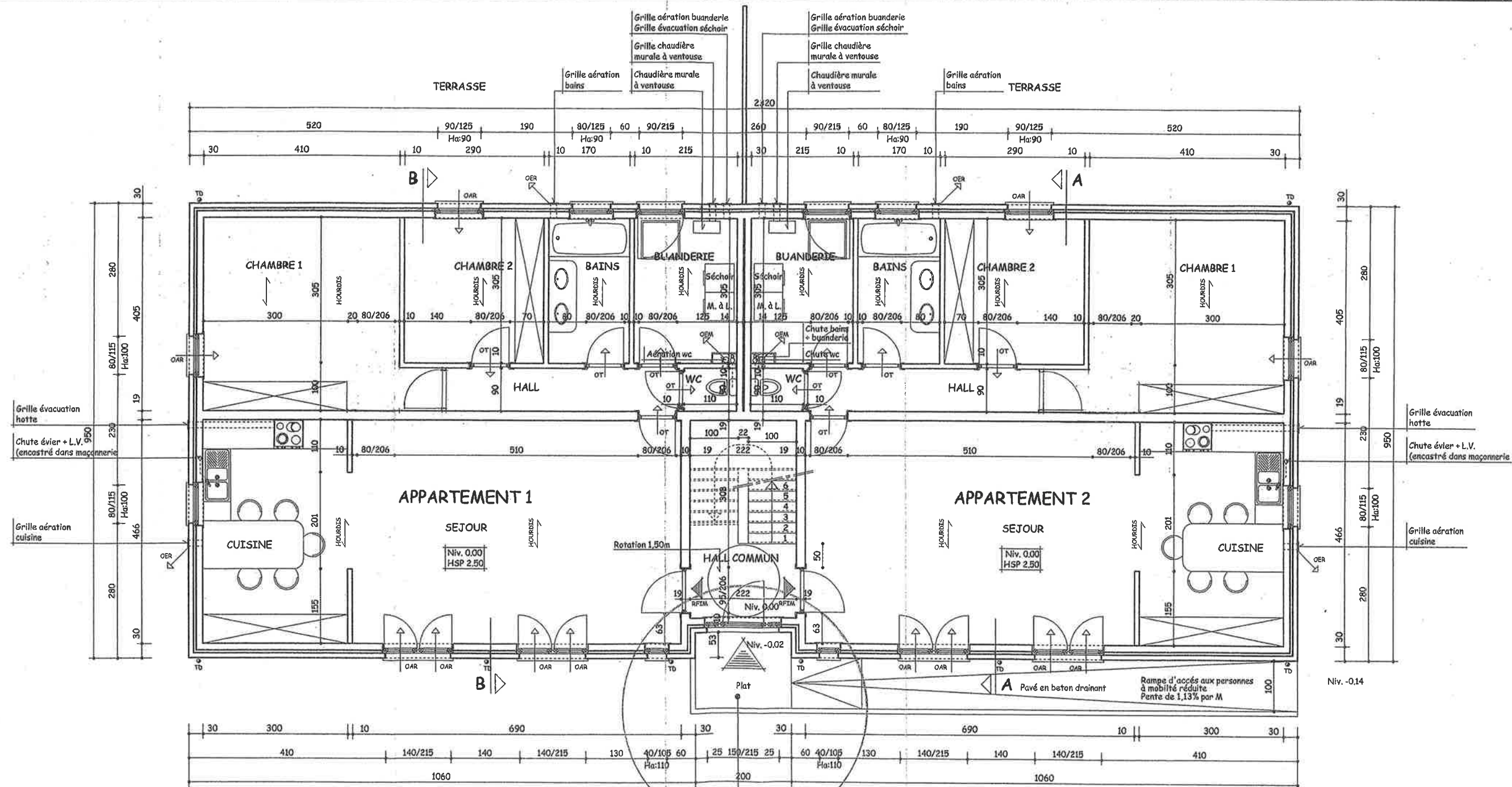
PLAN DU REZ-DE-CHAUSSEE
