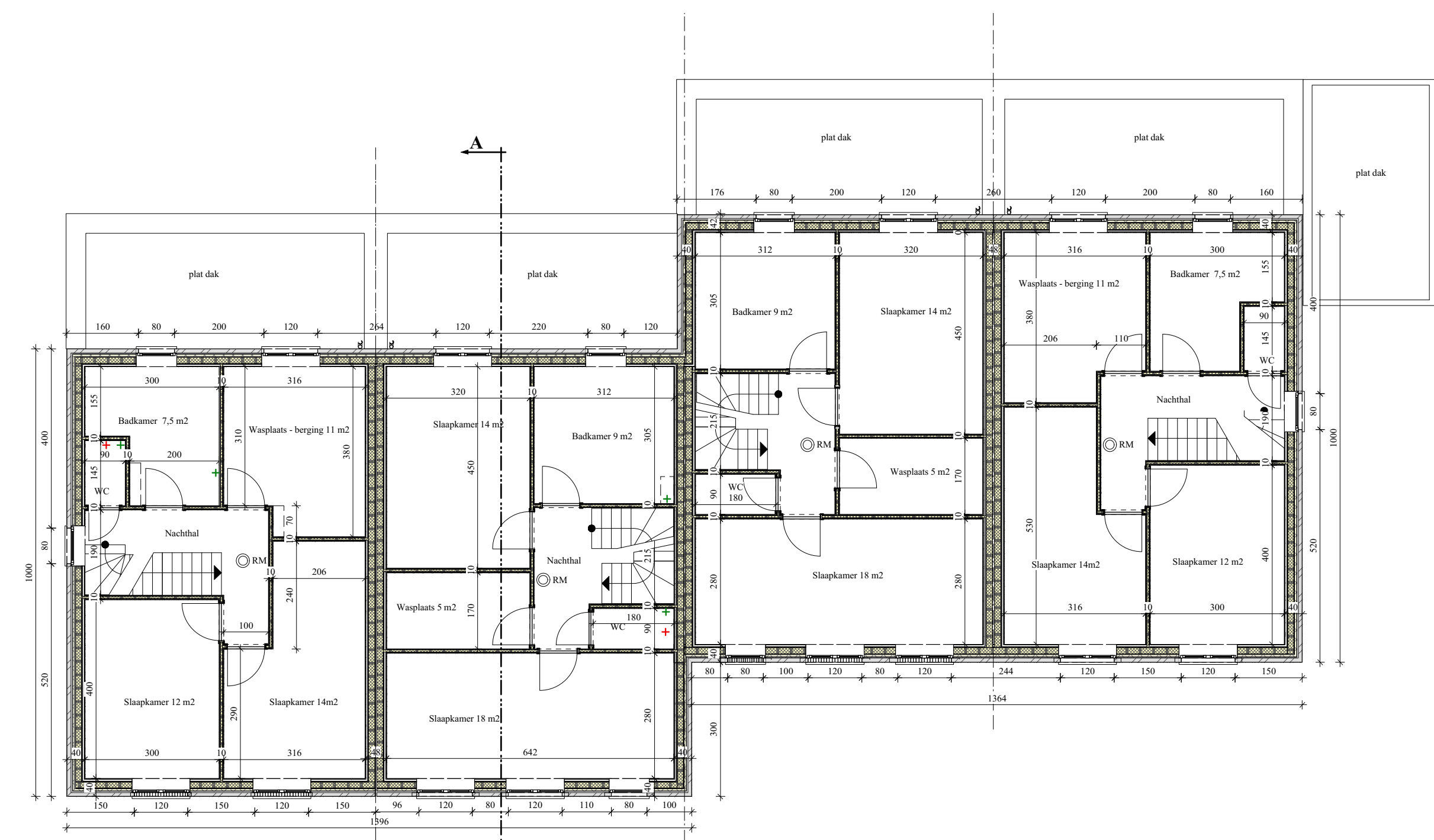
VERDIEPING
