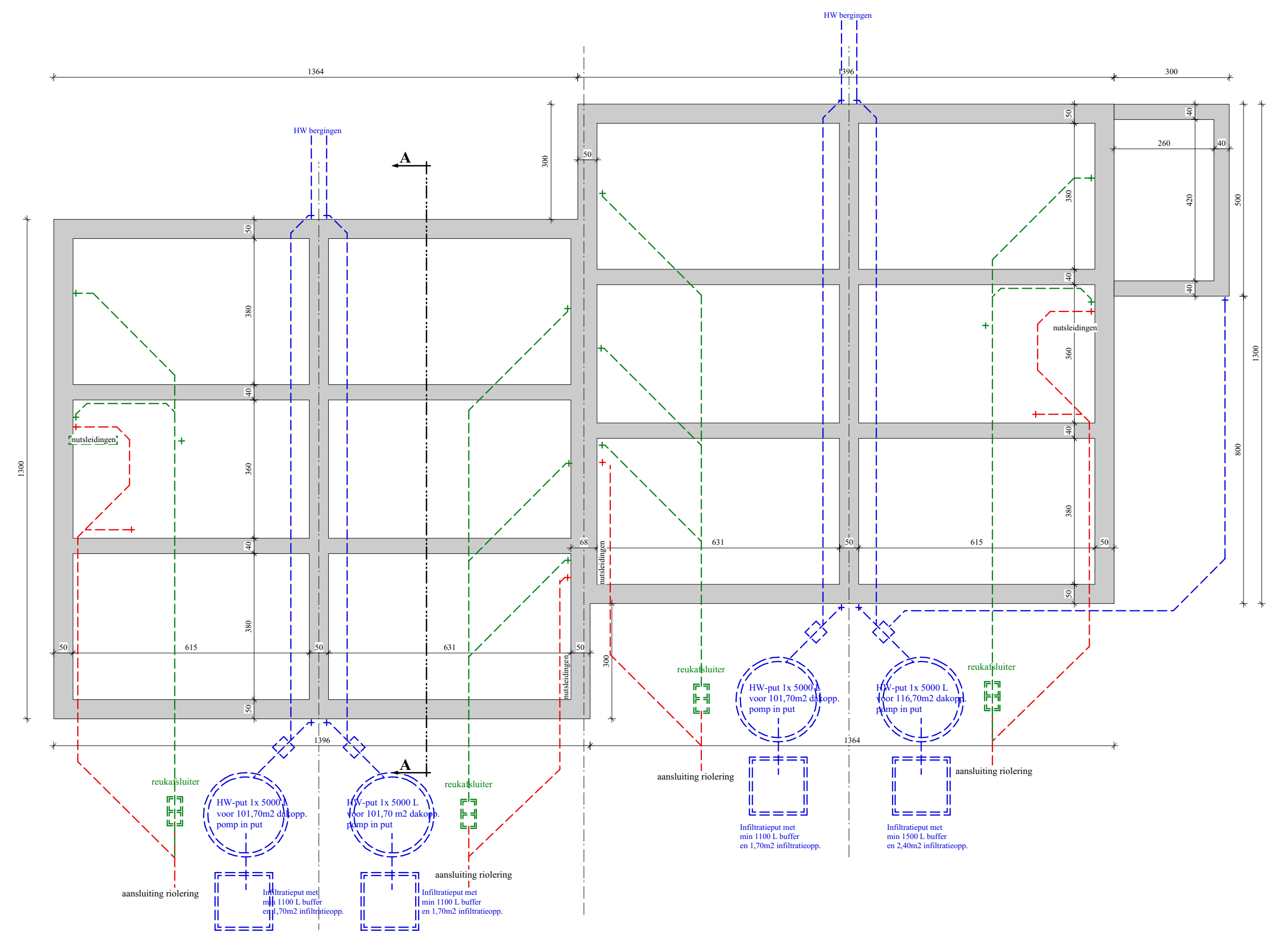
FUNDERING en RIOLERING
