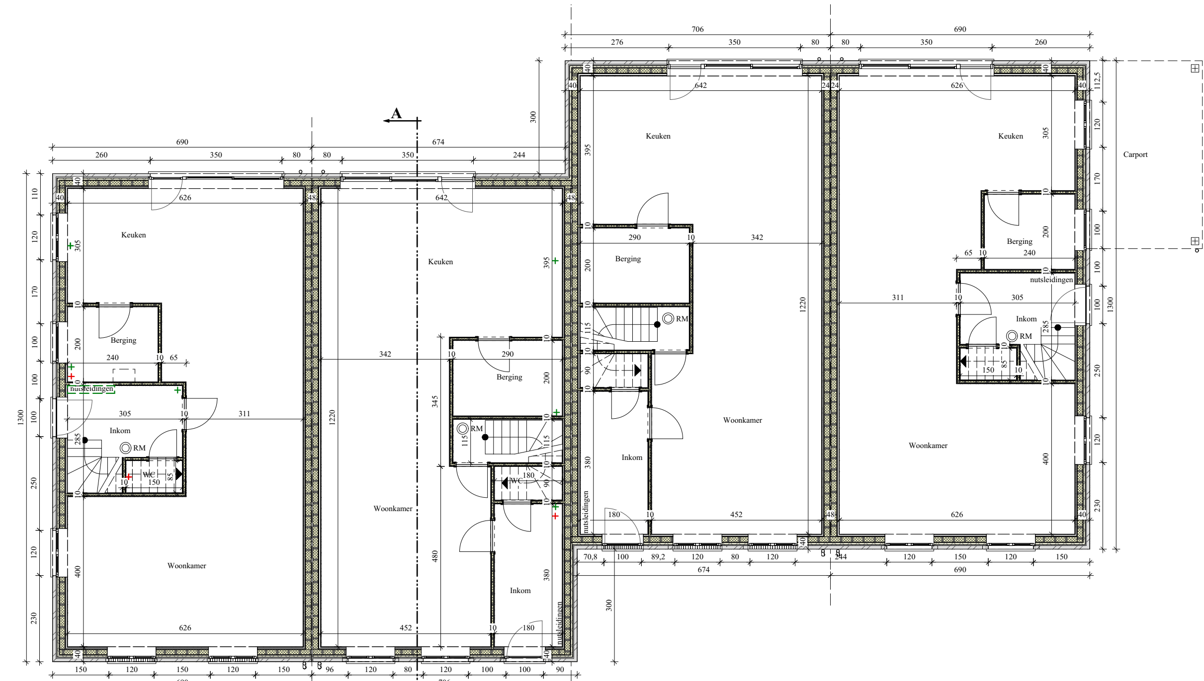
GELIJKVLOERS
