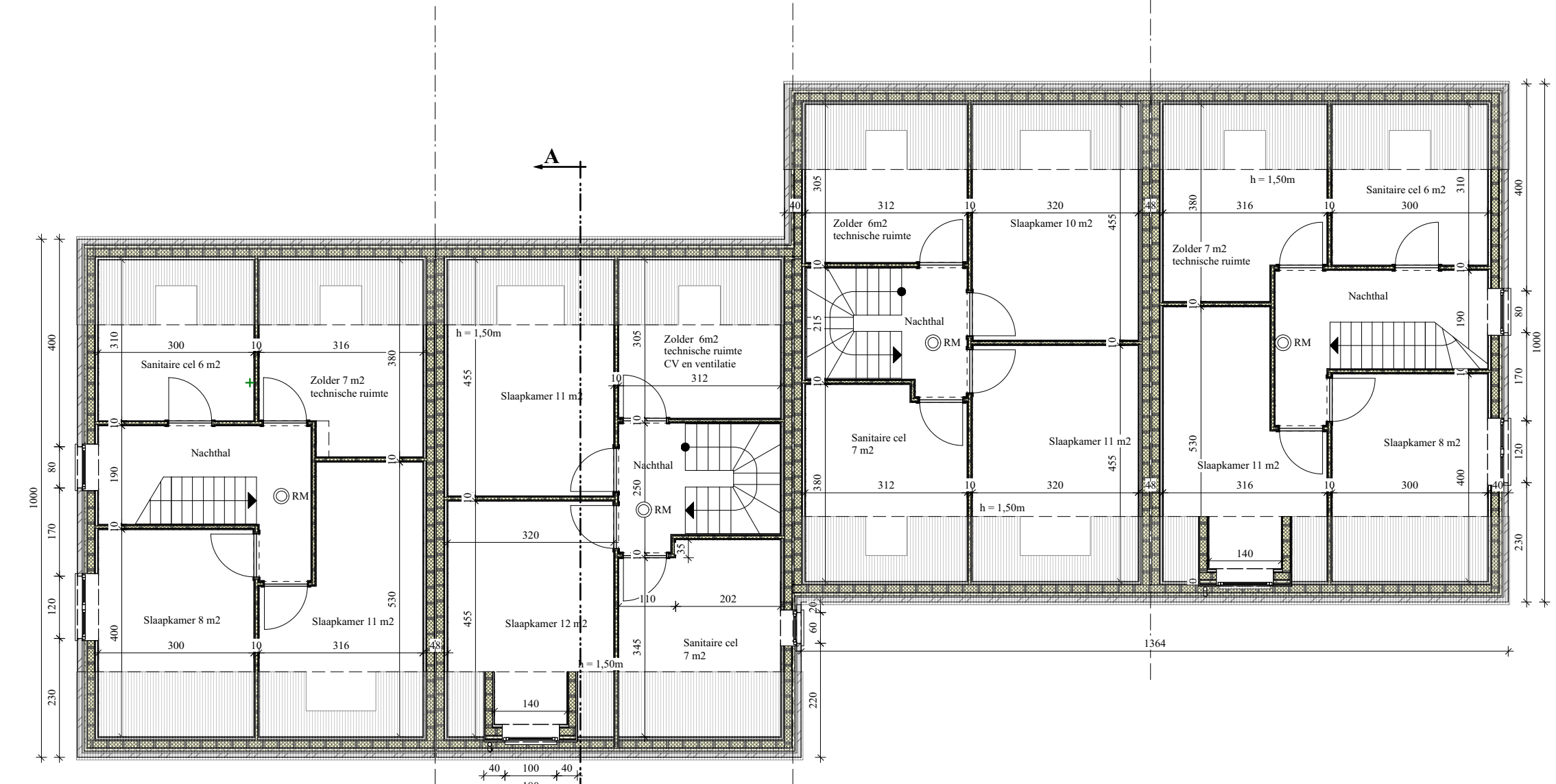
DAKVERDIEPING
