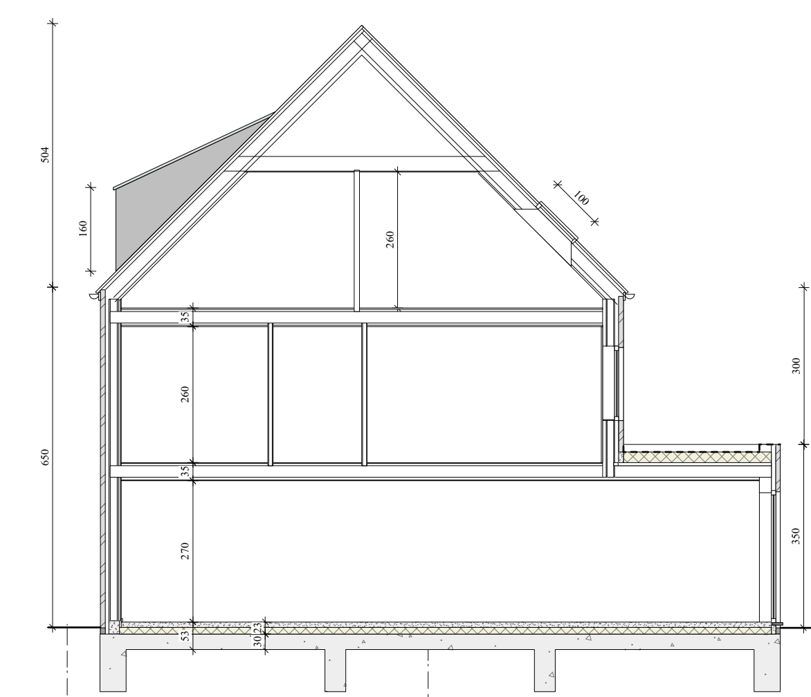
DOORSNEDE AA
