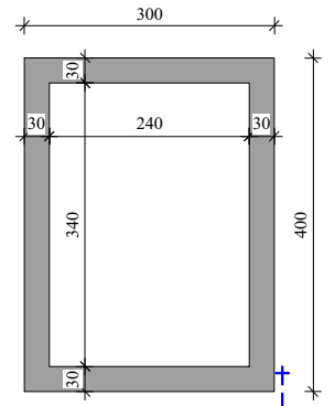
TUINBERGING fundering bij woning 3 en 4
