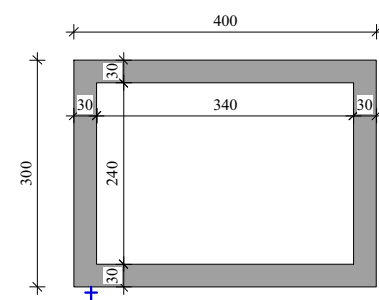
TUINBERGING fundering bij woning 1 en 2
