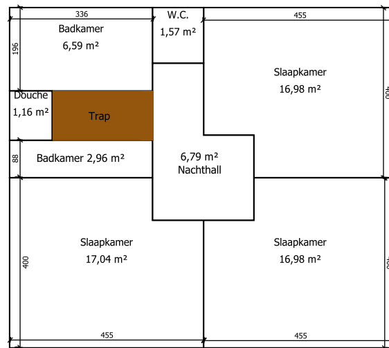
1ste verdieping
