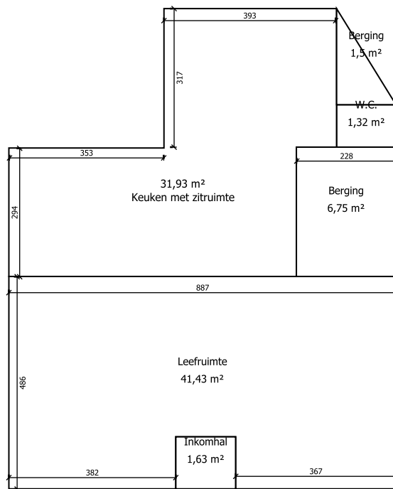
Gelijkvloers
