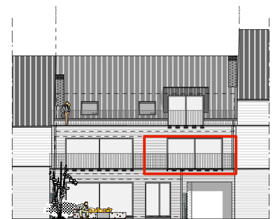
ACHTERGEVEL AANZICHT
